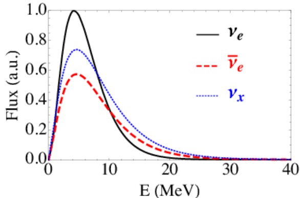
(d) ( g_{\text{ap}} = 9 \times 10^{-10}, \xi = 1 ) – PNS deleptonization phase
