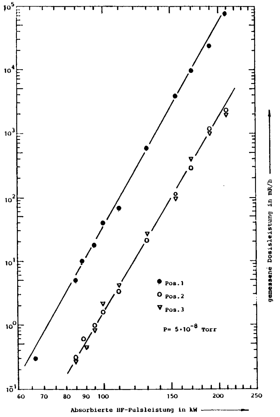
Abb. 2a Dosisleistung bei Pos. 1, 2 u. 3 an einem 5-Zeller. Das Tastverhältnis der absorbierten HF-Pulsleistung betrug 8,5%.
