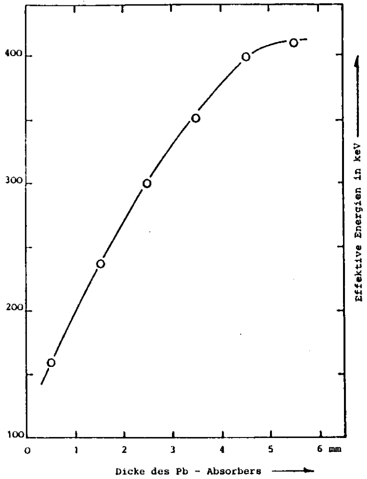
Abb.4 Effektive Energien für verschiedene Bleidicken.
