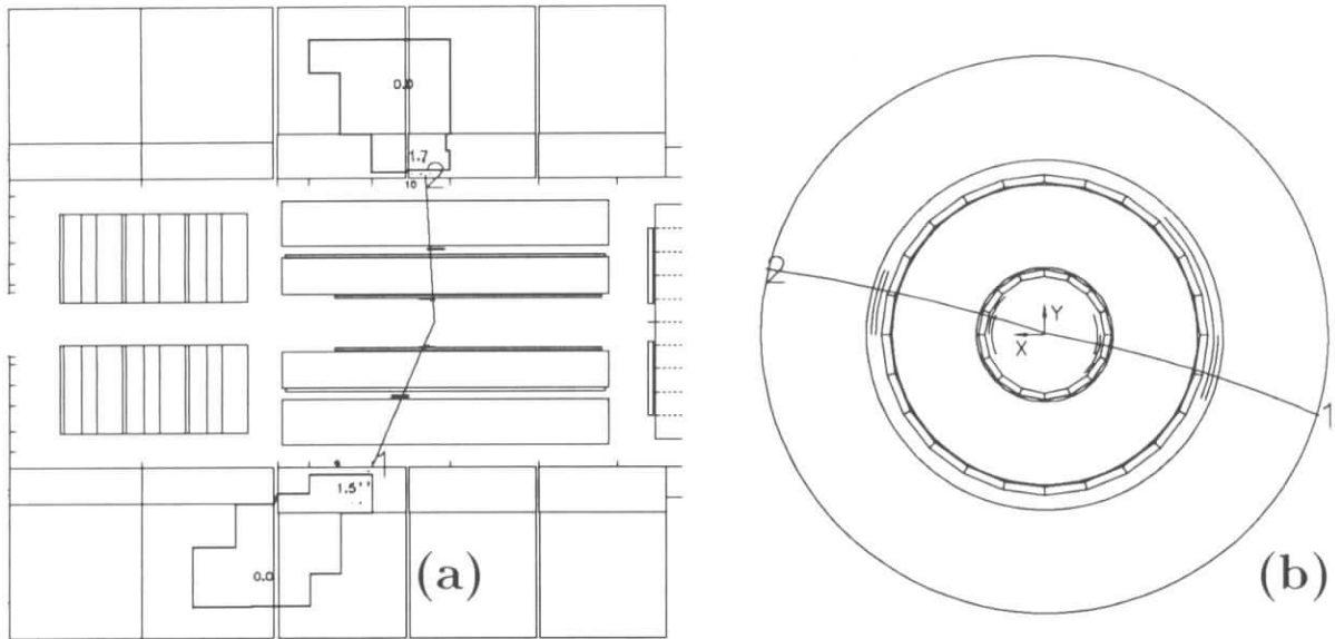
Abbildung 4.1: Abbildungen (a) und (b) erläutern die Funktionsweise des Triggers. (a) zeigt ein J/\psi \rightarrow e^+e^- -Ereignis in der rz -Ansicht. Das e^+e^- -Paar löst Signale in den Proportionalkammern aus, die die Ray-Information für den z -Vertex-Trigger liefern. Weiterhin sprechen die Segmente des Kalorimetertriggers an, die ein weiteres Triggererelement liefern. In (b) wird die MWPC-Information in der r\phi -Projektion gezeigt. Die beiden Spuren liegen koplunar zueinander. Dies löst das Triggererelement topo--BR aus.
