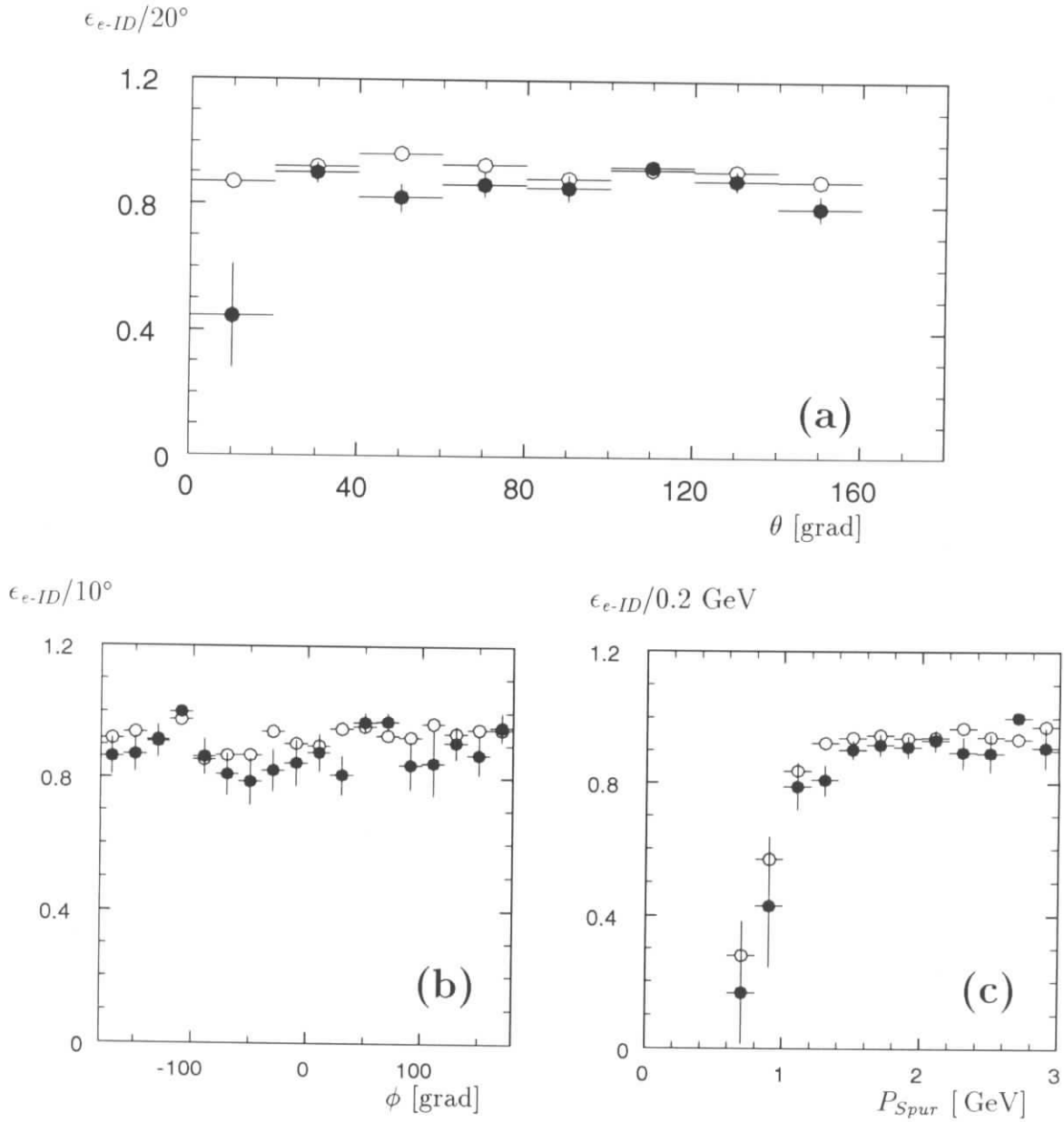
Abbildung 5.3: Elektronennachweiswahrscheinlichkeit in Abhängigkeit vom Polarwinkel (a), dem Azimutalwinkel (b) und dem Impuls (c) der Spur. Die ausgefüllten Punkte stehen für die Daten und die Kreise für die Monte-Carlo-Simulation.
