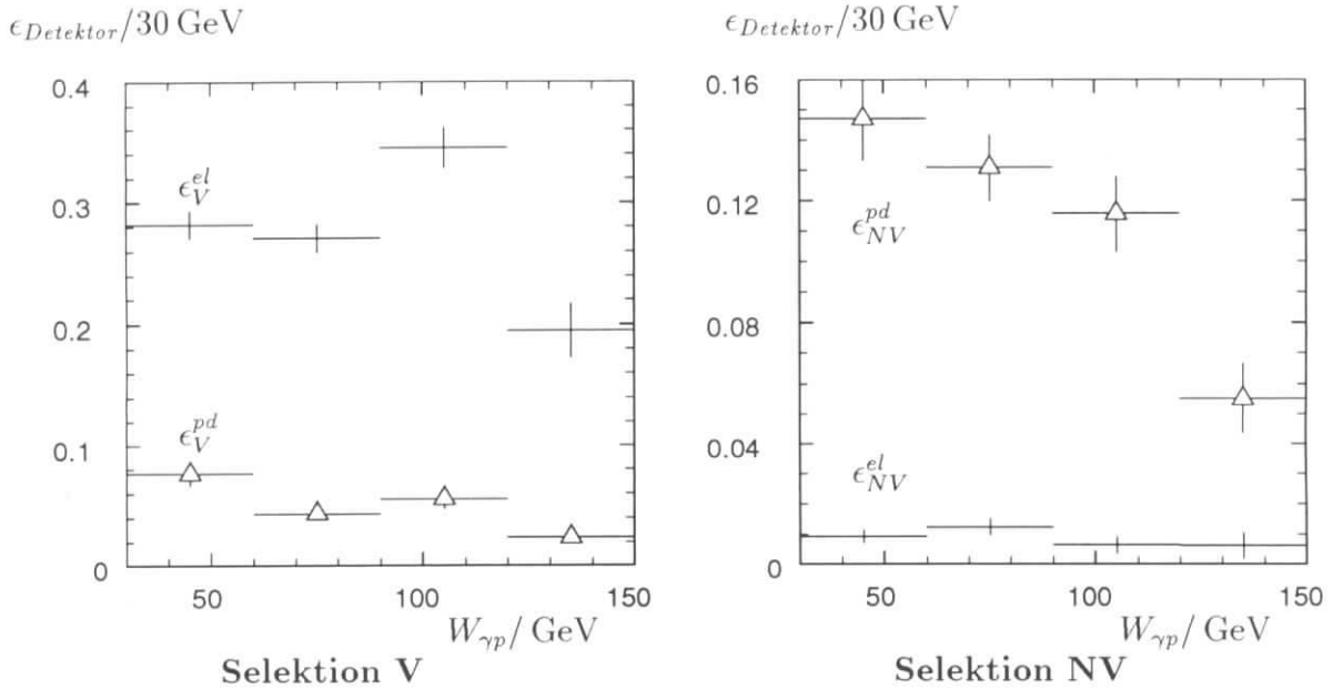
Abbildung 5.14: Detektorakzeptanz in Abhängigkeit von W_{\gamma p} getrennt für protonelastische und protoninelastische Ereignisse. Links sind die Akzeptanzen im Fall der Selektion V und rechts für die Selektion NV abgebildet. Das e^+e^- -Paar muß im Polarwinkelbereich zwischen 20^\circ < \theta < 160^\circ liegen und Q^2 < 4 \text{ GeV}^2 betragen. Der protonelastische Akzeptanzverlauf wird durch Balken und die protoninelastische Akzeptanz durch Dreiecke dargestellt.
