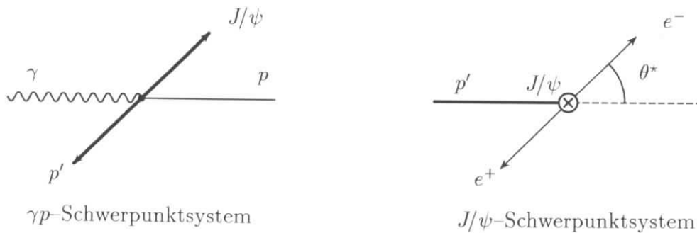
Abbildung 1.9: Darstellung des Zerfallswinkel \theta^* im J/\psi -Schwerpunktsystem. Als relevantes Bezugssystem dient das \gamma p -Schwerpunktsystem, welches die Quantisierungsachse für \theta^* definiert.
