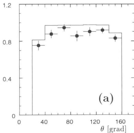
Abbildung 5.5: Abbildungen (a) und (b) zeigen jeweils die Nachweiswahrscheinlichkeiten für das Triggerelement dcrphi-tha des Driftkammertriggers. Das Monte-Carlo-Modell zeigt eine 8 % höhere Nachweiswahrscheinlichkeit als die Daten.
