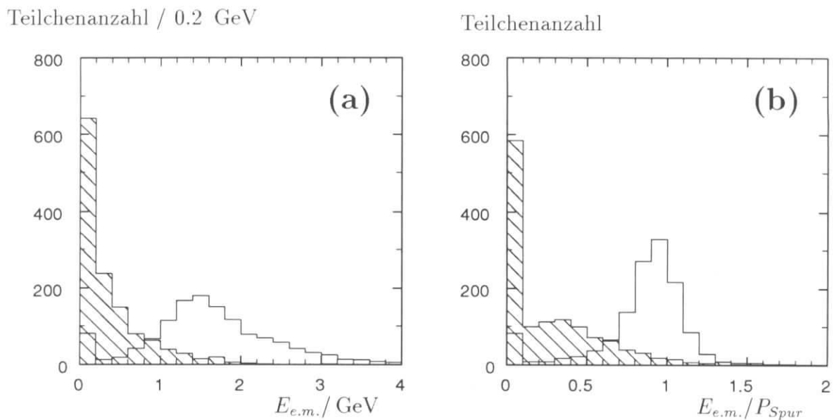
Abbildung 4.6: Vergleich zwischen Elektronen aus dem Zerfall des J/\psi -Mesons (Monte-Carlo-Modell) und Pionen aus Photoproduktionsdaten.
