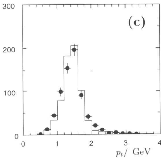
Abbildung 5.16: Die wichtigsten Verteilungen für die Spureigenschaften der Elektronen aus dem J/\psi -Zerfall. Die Daten sind als Punkte gekennzeichnet. Das Monte-Carlo-Modell nach allen Detektorschnitten ist als Histogramm überlagert. (Die Statistik des Monte-Carlo-Modells entspricht der fünffachen Statistik der Daten.)
