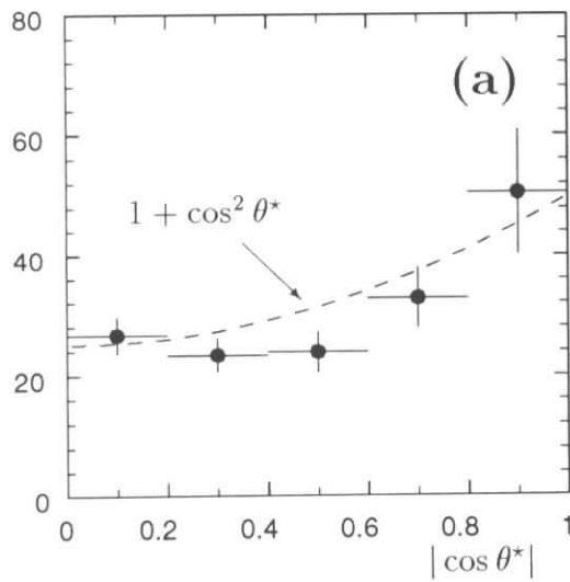
Abbildung 6.5: Abbildung (a): Auf Detektoreinflüsse korrigierte Zerfallswinkelverteilung im Vergleich zur Vorhersage transversal polarisierter J/\psi -Mesonen (Gleichung: 6.6). (b) zeigt für J/\psi -Mesonen die Polarakzeptanz nach dem Polarwinkelschnitt auf die beiden Zerfallsleptonen von 20^\circ < \theta < 160^\circ sowie die Detektorakzeptanz, die innerhalb des Polarwinkelbereichs ermittelt wurde.
