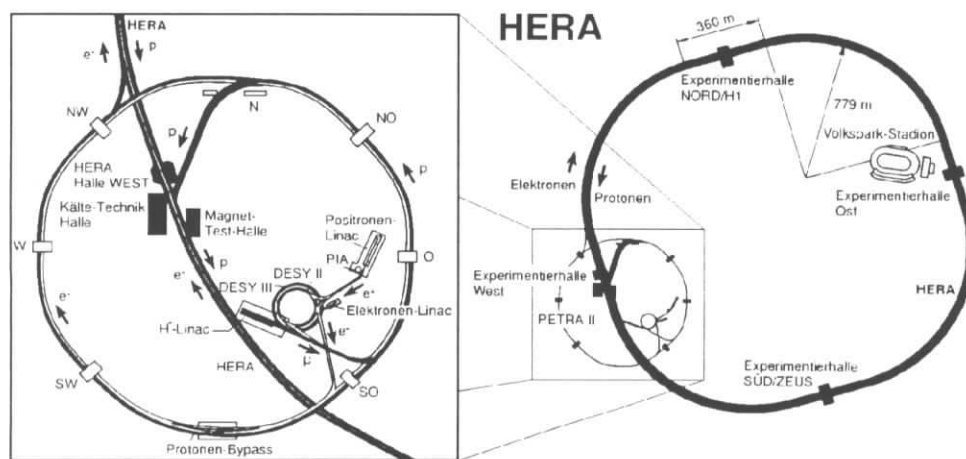
Abbildung 2.1: Die Speicherringanlage HERA und ihre Vorbeschleuniger
