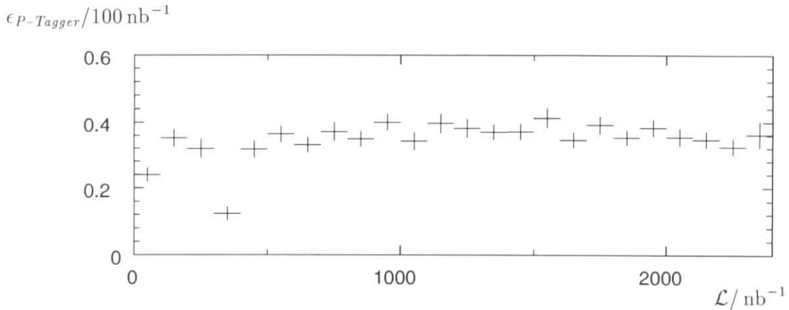
Abbildung 5.11: Relative Trefferhäufigkeit der Zählkanäle 0,1,3,5 des Proton-Taggers in Abhängigkeit von der Luminosität für das Ansprechen von mindestens einem Kanal.
