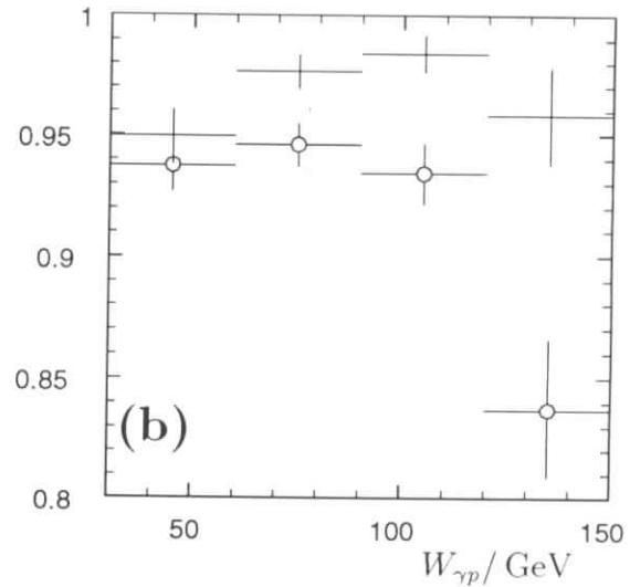
Abbildung 5.13: Abbildung (a) zeigt in Abhängigkeit von W_{\gamma p} die Akzeptanz für protoninelastische Ereignisse durch die Selektion NV , die Schauerpartikel aus der Protodissoziation nachweist. Abbildung (b) zeigt den Einfluß der Multiplizitätsbedingung, die nur die beiden Spuren des e^+e^- -Paares im Spurkammersystem zuläßt, auf den Nachweis von protoninelastischen Ereignissen. Im Monte-Carlo-Modell wird der Fall n = 2 durch Punkte mit Kreisen und n = 2.5 durch die Balken dargestellt.
