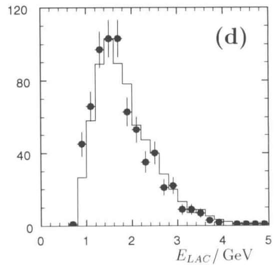
Abbildung 5.16: Die wichtigsten Verteilungen für die Spureigenschaften der Elektronen aus dem J/\psi -Zerfall. Die Daten sind als Punkte gekennzeichnet. Das Monte-Carlo-Modell nach allen Detektorschnitten ist als Histogramm überlagert. (Die Statistik des Monte-Carlo-Modells entspricht der fünffachen Statistik der Daten.)
