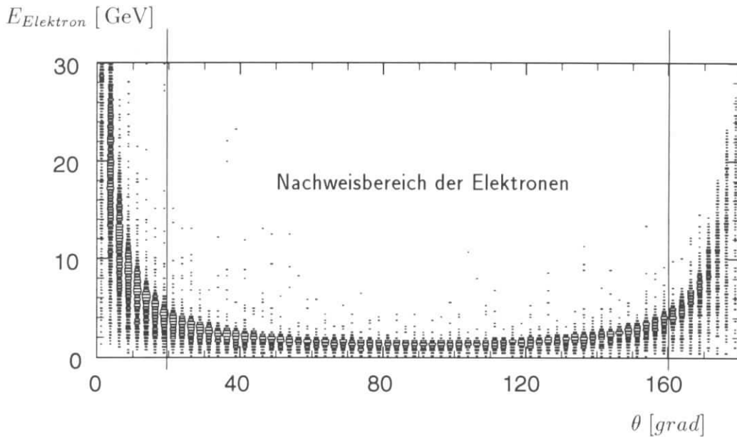
Abbildung 3.2: Energieverteilung der Elektronen aus dem Zerfall des J/\psi -Mesons in Abhängigkeit vom Polarwinkel \theta im Laborsystem. Die senkrechten Markierungen geben den Schnitt im Polarwinkelbereich zum Nachweis der Elektronen im Detektor an.
