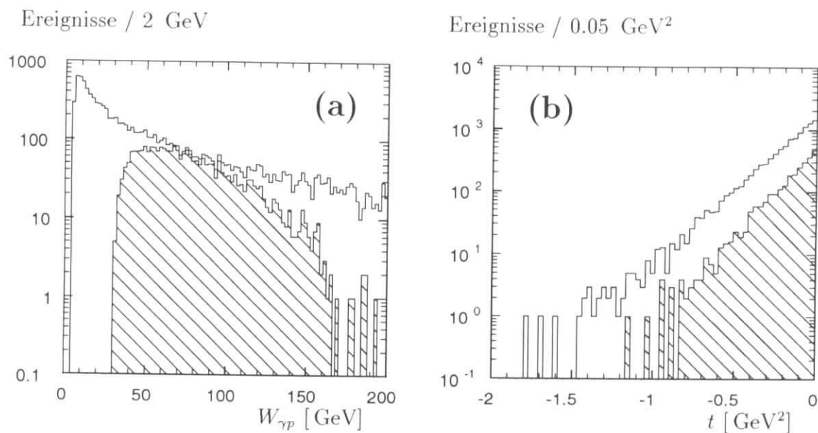
Abbildung 3.3: Abbildung (a) zeigt W_{\gamma p} vor und nach Einschränkung des Polarwinkelbereichs (schraffiert) für das Elektron-Positron-Paar. In (b) ist die t -Verteilung des elastischen Monte-Carlo-Generators dargestellt.
