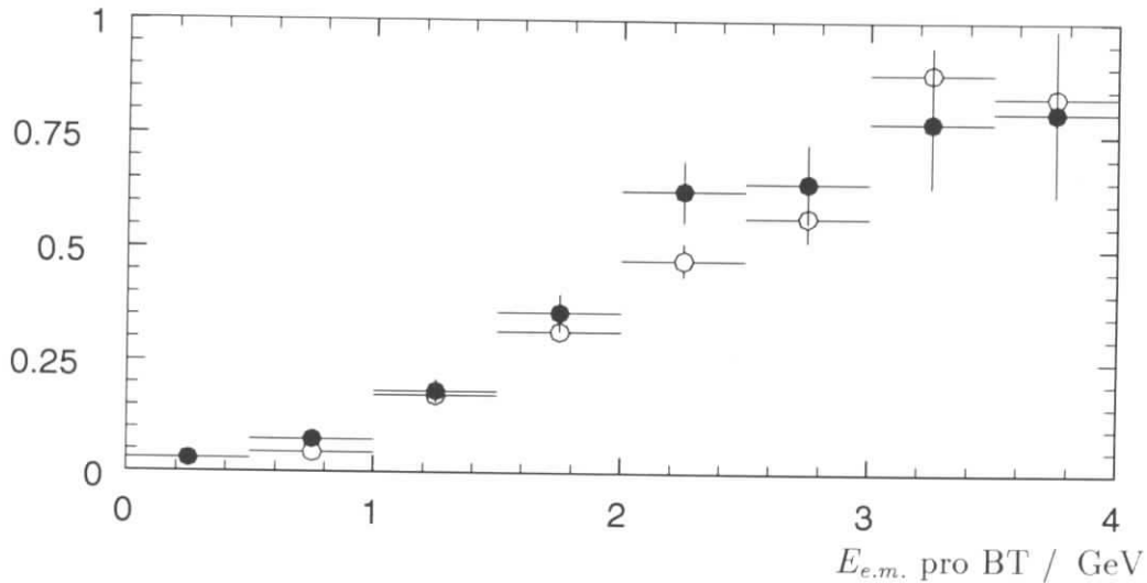
Abbildung 5.7: Das Ansprechverhalten eines Big-Towers in Abhängigkeit von der elektromagnetischen Energie, die in diesem Big-Tower deponiert wurde. In dieser Abbildung werden das Verhalten im Monte-Carlo-Modell (Kreise) mit den Daten (ausgefüllte Punkte) verglichen.
