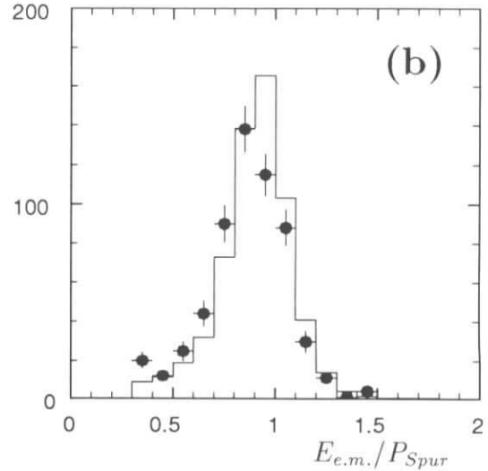
Abbildung 5.2: Abbildung (a) zeigt die rekonstruierte Energie im LAC im direkten Vergleich zwischen Daten (Punkte) und Monte-Carlo-Simulation (Histogramm). In (b) ist das E/P -Verhältnis dargestellt.
