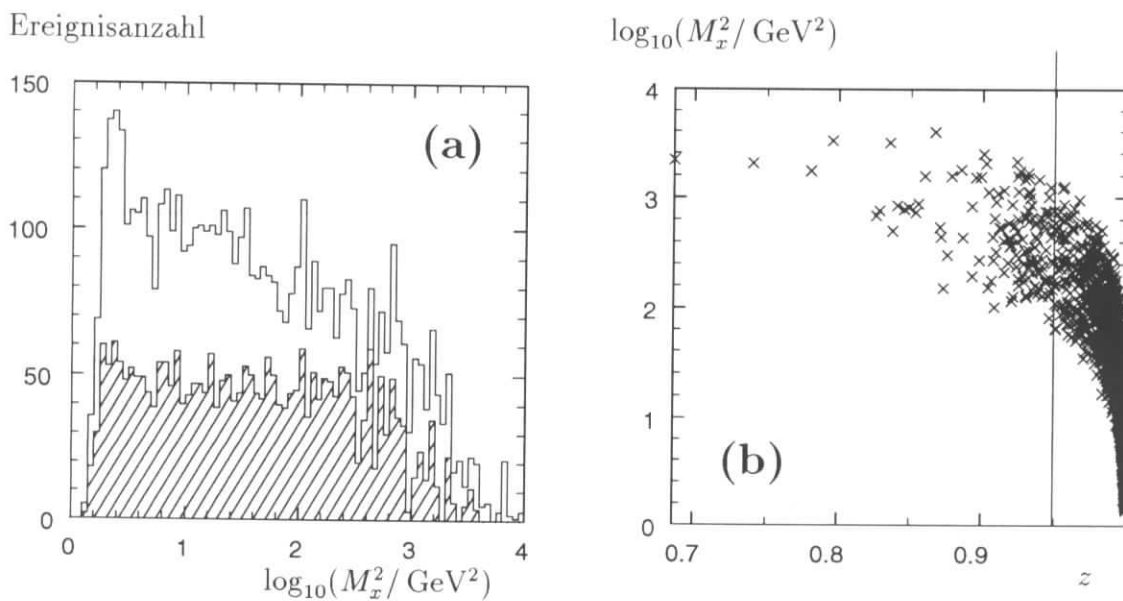
Abbildung 3.4: In Abbildung (a) wird die M_x^2 -Verteilung vor und nach dem Polarwinkelschnitt gezeigt. In (b) ist die Korrelation zwischen der z -Verteilung und M_x^2 nach dem Polarwinkelschnitt dargestellt. Mit einem Schnitt von z > 0.95 läßt sich die Protodissoziation nicht vollständig unterdrücken.
