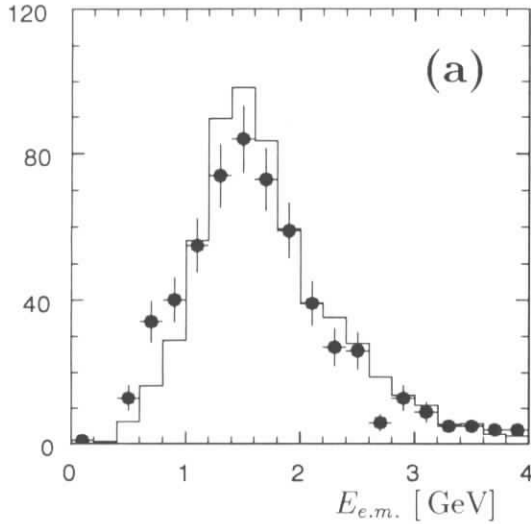
Abbildung 5.2: Abbildung (a) zeigt die rekonstruierte Energie im LAC im direkten Vergleich zwischen Daten (Punkte) und Monte-Carlo-Simulation (Histogramm). In (b) ist das E/P -Verhältnis dargestellt.
