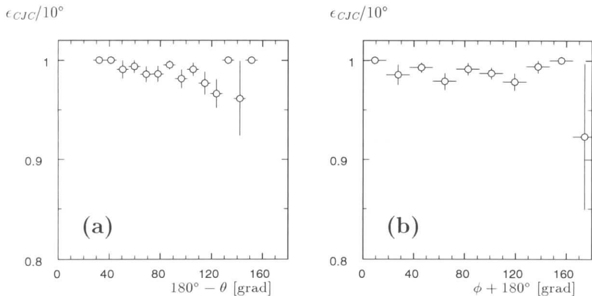
Abbildung 5.1: Nachweiswahrscheinlichkeit einer Spur im CJC-Spurkammersystem ermittelt durch kosmische Myonen: Abbildung (a) zeigt die Abhängigkeit vom Polarwinkel. (b) zeigt den Azimutalbereich.
