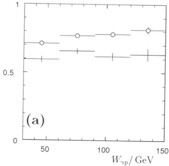
Abbildung 5.13: Abbildung (a) zeigt in Abhängigkeit von W_{\gamma p} die Akzeptanz für protoninelastische Ereignisse durch die Selektion NV , die Schauerpartikel aus der Protodissoziation nachweist. Abbildung (b) zeigt den Einfluß der Multiplizitätsbedingung, die nur die beiden Spuren des e^+e^- -Paares im Spurkammersystem zuläßt, auf den Nachweis von protoninelastischen Ereignissen. Im Monte-Carlo-Modell wird der Fall n = 2 durch Punkte mit Kreisen und n = 2.5 durch die Balken dargestellt.
