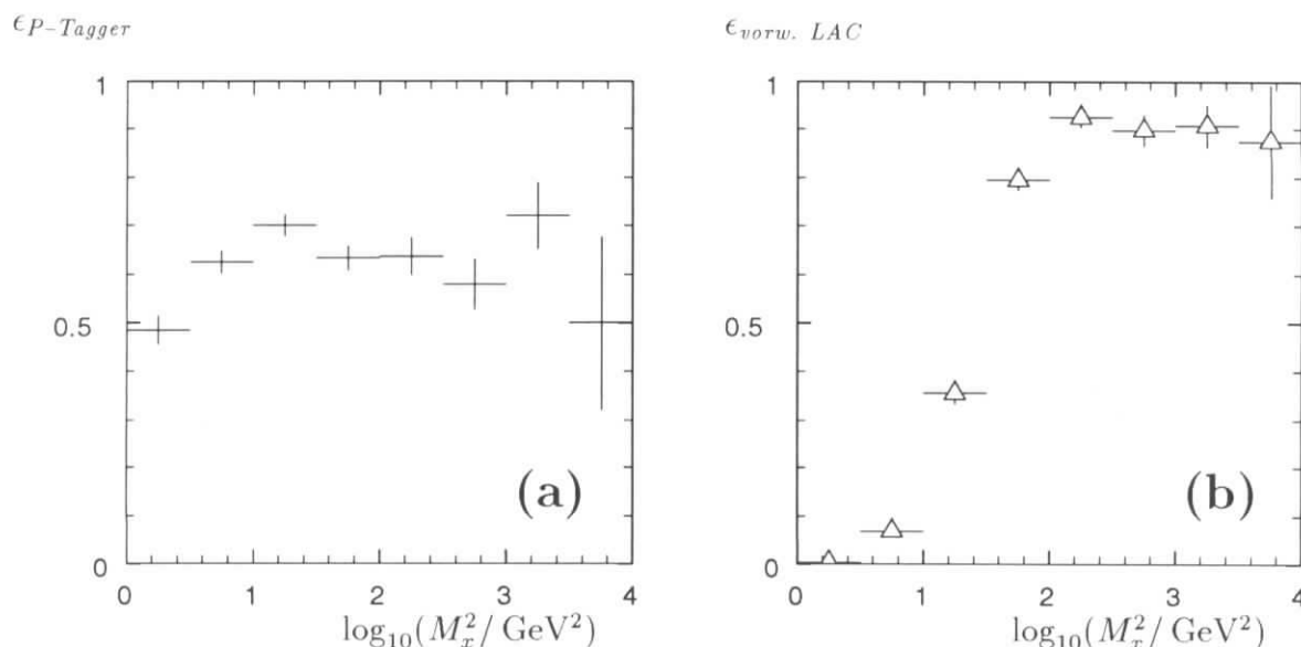
Abbildung 5.12: Abbildung (a) zeigt die Akzeptanz des Proton-Taggers und Abbildung (b) des LAC-Kalorimeters mit E_{IF} > 1 \text{ GeV}^2 in Abhängigkeit von \log_{10}(M_x^2 / \text{GeV}^2) , für das Monte-Carlo mit Protodissoziation.
