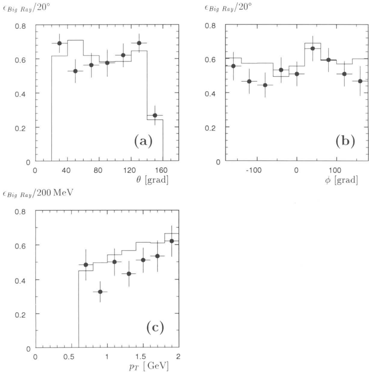
Abbildung 5.6: Die Ansprechwahrscheinlichkeit für Big-Ray-Signale in Abhängigkeit vom Winkelbereich (a), (b) nach dem Durchgang einer Spur durch das zugehörige räumliche Proportionalkammersegment. Abbildung (c) zeigt das Ansprechverhalten der Proportionalkammersegmente in Abhängigkeit vom Transversalimpuls der Spur. Für die Daten (Punkte) und die Monte-Carlo-Ereignisse wurde die Selektion nach Tabelle 5.3 durchgeführt. Die Monte-Carlo-Simulation ist als Histogramm überlagert dargestellt.
