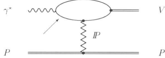
Abbildung 1.8: Diagramm für \gamma^* p \rightarrow V p bei großem Q^2 . Die mit dem Pfeil gekennzeichnete Quarklinie ist weit von der Massenschale entfernt (Abb. aus [Don87]).
