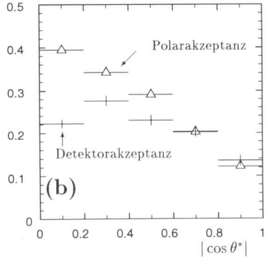
Abbildung 6.5: Abbildung (a): Auf Detektoreinflüsse korrigierte Zerfallswinkelverteilung im Vergleich zur Vorhersage transversal polarisierter J/\psi -Mesonen (Gleichung: 6.6). (b) zeigt für J/\psi -Mesonen die Polarakzeptanz nach dem Polarwinkelschnitt auf die beiden Zerfallsleptonen von 20^\circ < \theta < 160^\circ sowie die Detektorakzeptanz, die innerhalb des Polarwinkelbereichs ermittelt wurde.
