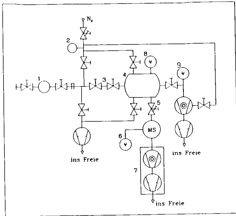
Abbildung 4.2: 1: Probenkugel mit Ventilen, 2: Ballon, 3: Schleuse, 4: Expansionskessel, 5: Metallschneidventil, 6: Penningmanometer, 7: automatischer Pumpstand, 8: Thermotransmanometer, 9: Penningmanometer
