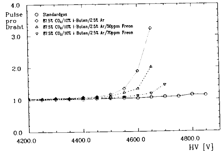
Abbildung 6.8: Mittlere Anzahl der Pulse auf einem Draht in Abhängigkeit von der Hochspannung. Gemittelt wurde über alle Drähte mit mindestens einem Puls über 50mV.
