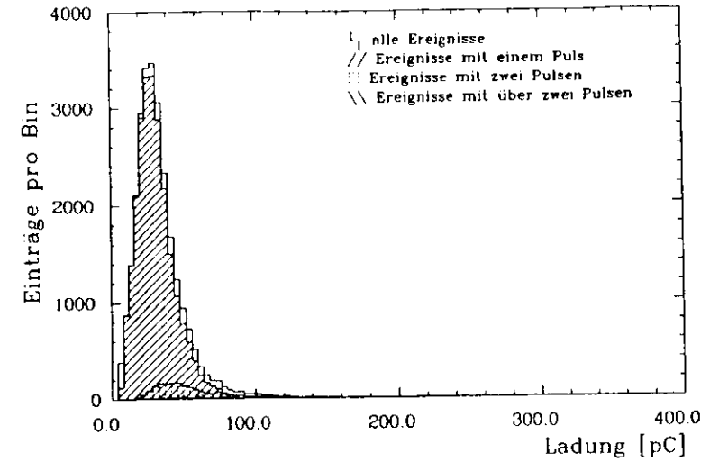
Abbildung 6.4: Häufigkeitsverteilung der Streamerladung für das Standardgas (25% Argon, 75% Isobutan) bei einer Betriebsspannung von 4650V
