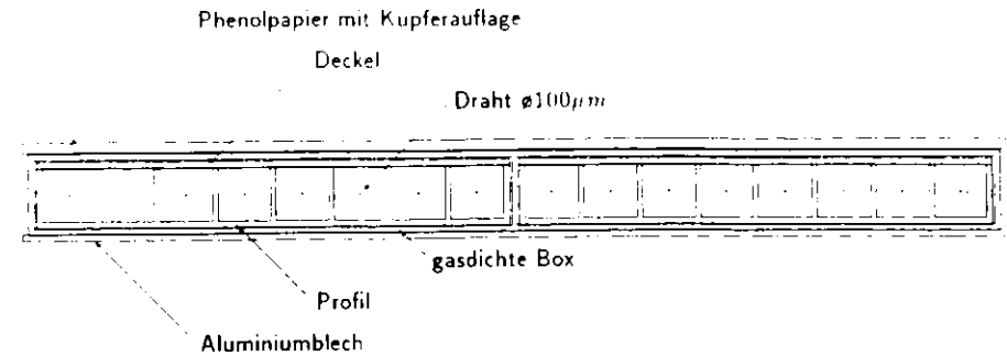
Abbildung 3.1: Querschnitt durch ein H1-Streamerrohr-Element in Originalgröße
