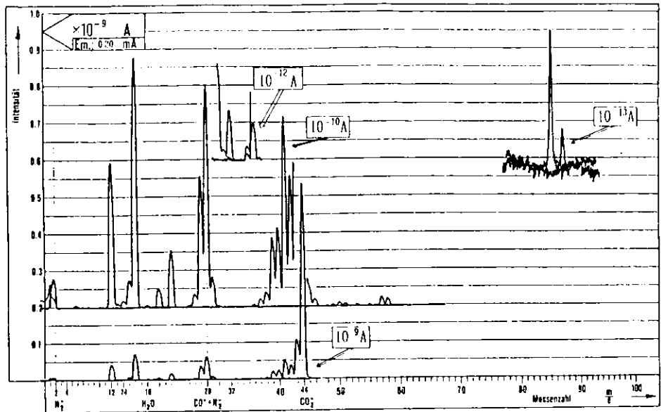
Abbildung 4.3: Massespektrum des nichtbrennbaren Gases mit 70ppm Freon (87,5% CO 2 , 10% Isobutan, 2,5% Argon, 70ppm Freon 114). Der Druck im Quadrupolmassenspektrometer betrug 2,5 \cdot 10^{-5} hPa .
