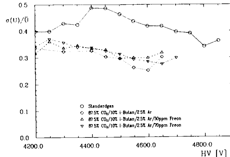
Abbildung 6.11: Relative Breiten der Pulshöhenverteilungen aller Pulse über 50mV in Abhängigkeit von der Hochspannung
