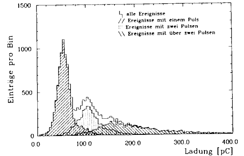
Abbildung 6.5: Häufigkeitsverteilung der Streamerladung für das nichtbrennbare Gas ohne Freon (2.5% Argon, 87.5% CO 2 , 10% Isobutan) bei einer Betriebsspannung von 46001V
