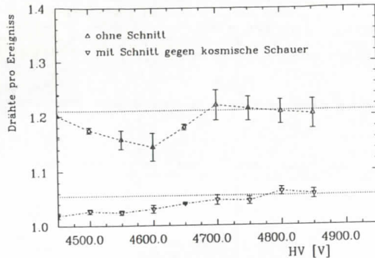
Abbildung 6.2: Mittlere Anzahl der Drähte mit Pulsen über 50mV für das Standardgas in Abhängigkeit von der Hochspannung. Es muß mindestens ein Draht ansprechen.
