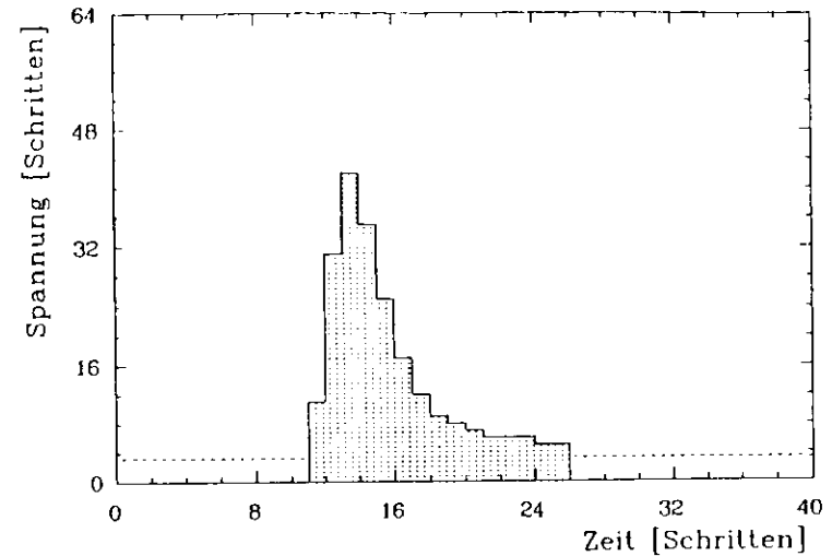
Abbildung 3.5: Puls und Pedestal bestimmt durch den Pulsfindalgorithmus während der Datennahme
