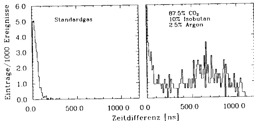
Abbildung 6.18: Zeitdifferenz zwischen erstem Drahtpuls und erstem Puls auf einem Nachbardraht bei einer Betriebsspannung 4650V
