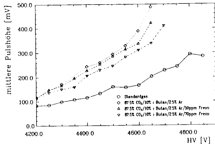
Abbildung 6.10: Mittlere Pulshöhe aller Pulse über 50mV in Abhängigkeit von der Hochspannung
