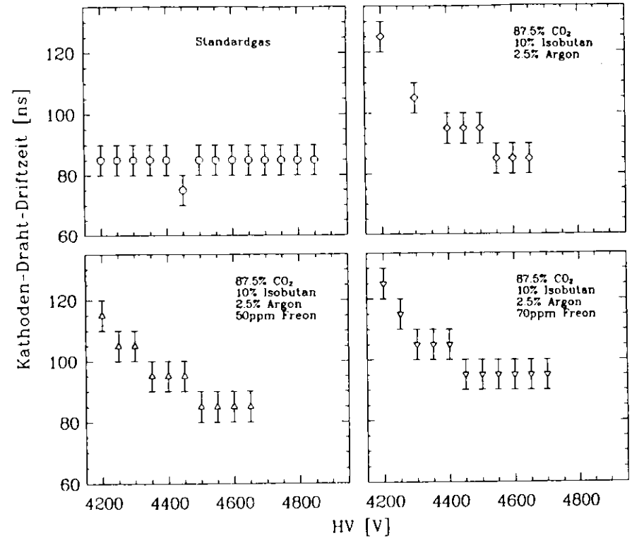
Abbildung 6.13: Die Kathoden-Draht-Driftzeit, ermittelt durch die Anzahl der Zeitscheiben, die 90% der Pulsmaxima enthalten, in Abhängigkeit von der Hochspannung
