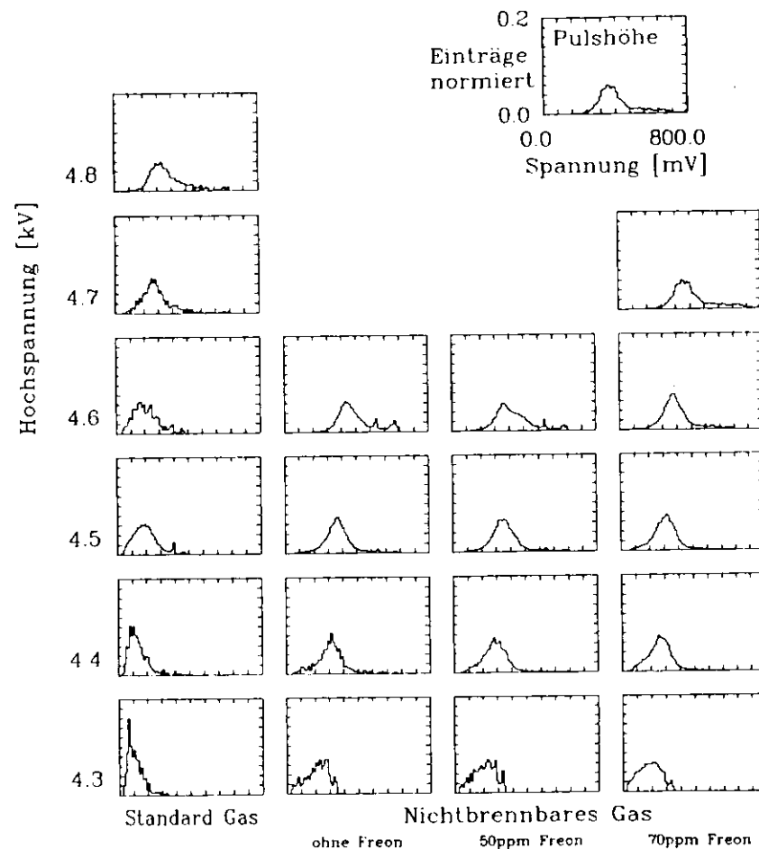
Abbildung 6.9: Häufigkeitsverteilungen der Pulshöhen für verschiedene Gase und Betriebsspannungen
