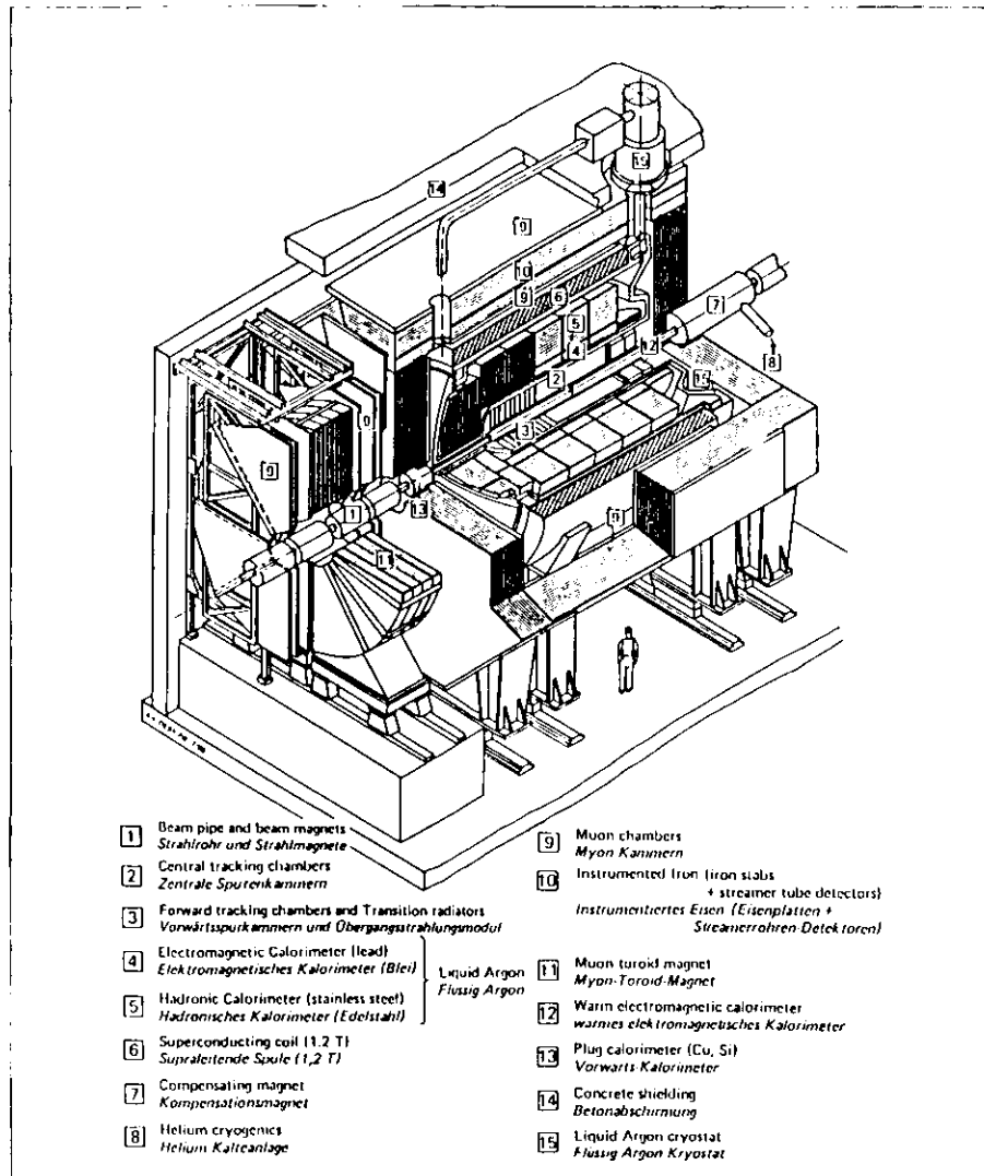
Abbildung 1.1: Der Aufbau des H1-Detektors [2]
