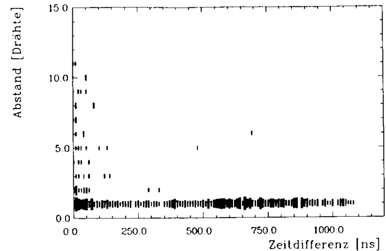
Abbildung 6.16: Korrelation zwischen der Zeitdifferenz und der Differenz der Drahtnummer für nichtbrennbares Gas ohne Freon bei 4650V
