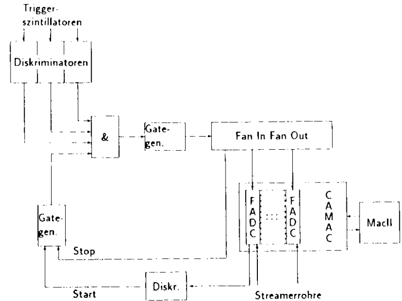
Abbildung 3.3: Blockschaltbild der Auslesesteuerung
