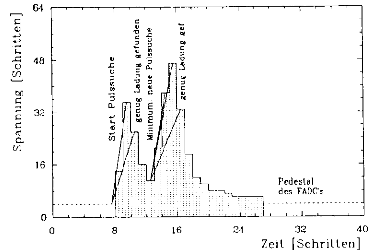
Abbildung A.1: Ein Beispiel für die Suche nach Mehrfachpulsen
