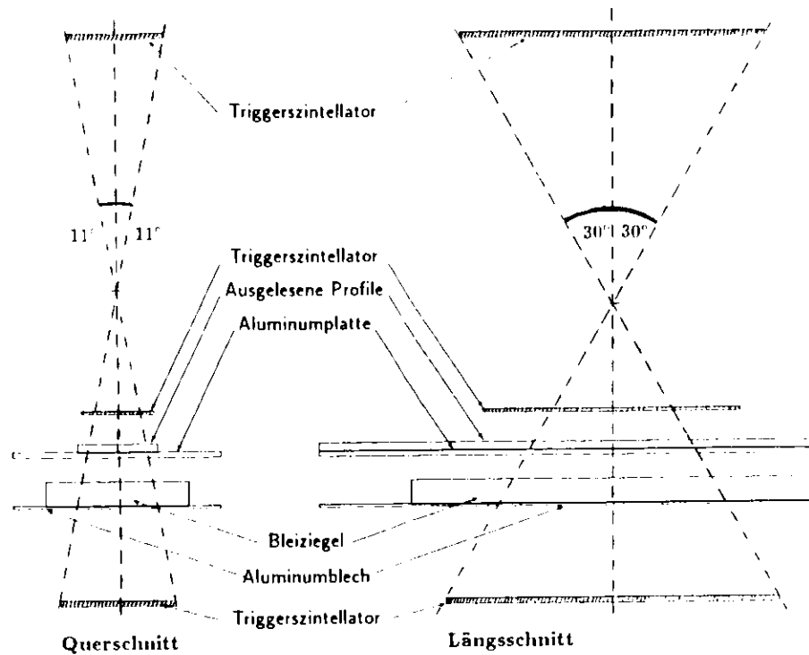
Abbildung 3.2: Querschnitt und Längsschnitt durch den Triggeraufbau, Maßstab 10:1
