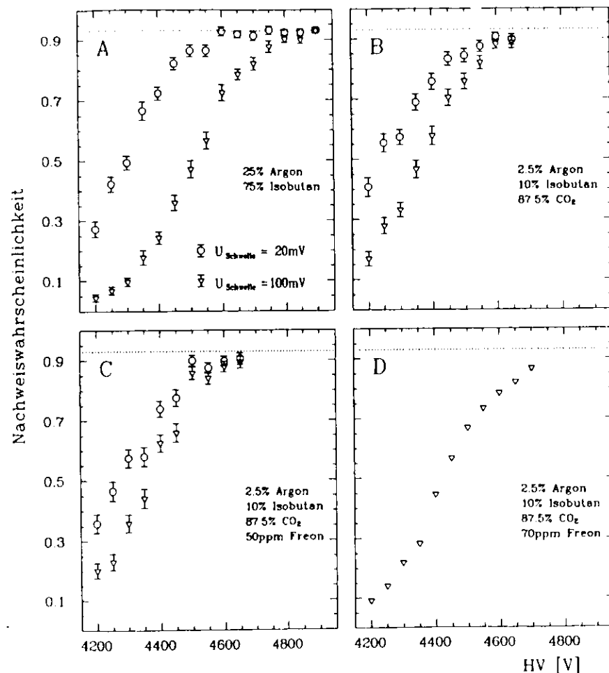
Abbildung 6.1: Nachweiswahrscheinlichkeit für alle untersuchten Gase in Abhängigkeit von der Hochspannung
