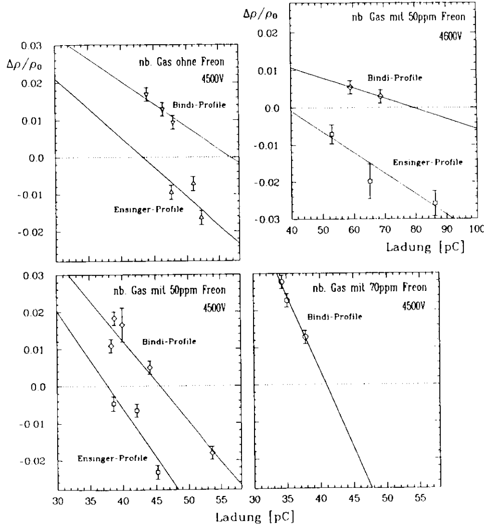
Abbildung 6.19: Die Abhängigkeit der Streamerladung von der Dichte für die nichtbrennbaren Gase
