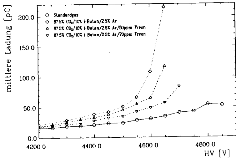
Abbildung 6.6: Mittlere Ladung aller Ereignisse mit mindestens einem Puls über 50mV in Abhängigkeit von der Hochspannung
