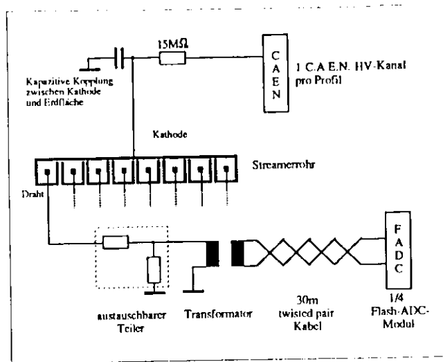
Abbildung 3.4: Schaltbild für die Auslese der Drähte und die Hochspannungsversorgung
