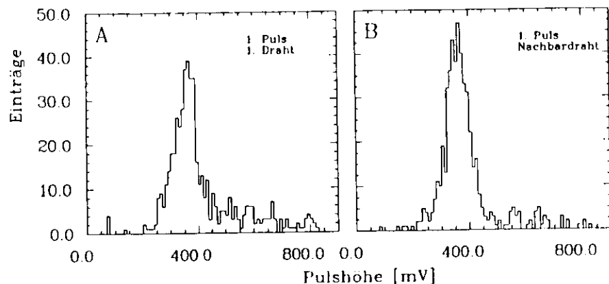
Abbildung 6.17: Die Pulshöhen für nichtbrennbares Gas ohne Freon und 4650V. Es wurden nur Ereignisse eingetragen, bei denen auch ein Nachbardraht des jeweils frühesten Drahtes anspricht.
