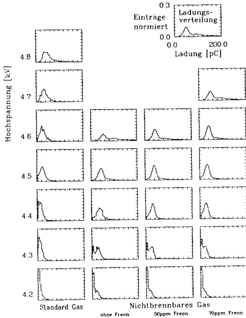
Abbildung 6.3: Häufigkeitsverteilungen der Streamerladungen für verschiedene Gase und Betriebsspannungen
