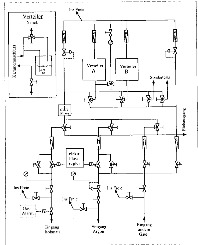
Abbildung 3.6: Schaltbild der verwendeten Gasmischanlage
