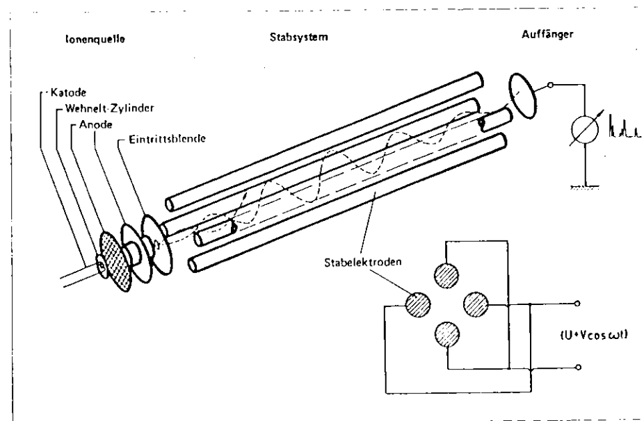
Abbildung 4.1: Schematischer Aufbau des QMA 112 [12]
