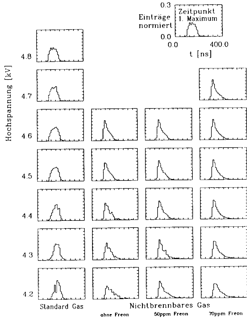
Abbildung 6.12: Häufigkeitsverteilungen der Zeitpunkte für das erste Pulsmaximum bei verschiedenen Gasen und Betriebsspannungen (Driftzeitverteilungen)
