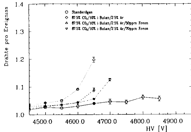
Abbildung 6.15: Mittlere Anzahl der Drähte mit Pulsen über 50mV nach dem Schnitt gegen kosmische Schauer. Es muß mindestens ein Draht ansprechen.
