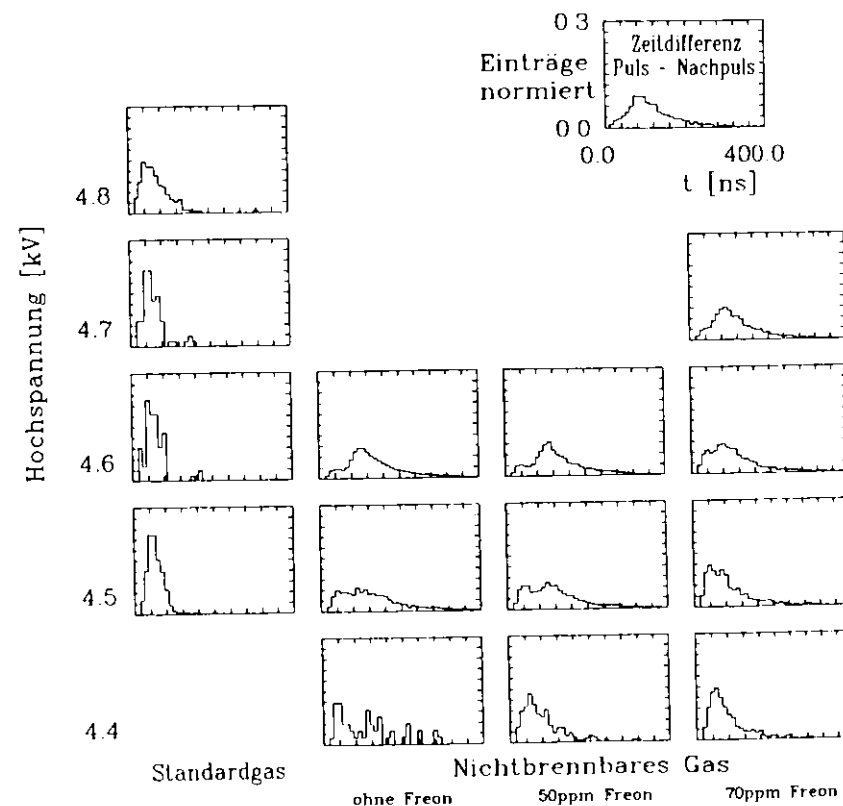
Abbildung 6.14: Häufigkeitsverteilungen der Zeitdifferenzen zwischen den Pulsen auf einem Draht für verschiedene Gase und Betriebsspannungen
