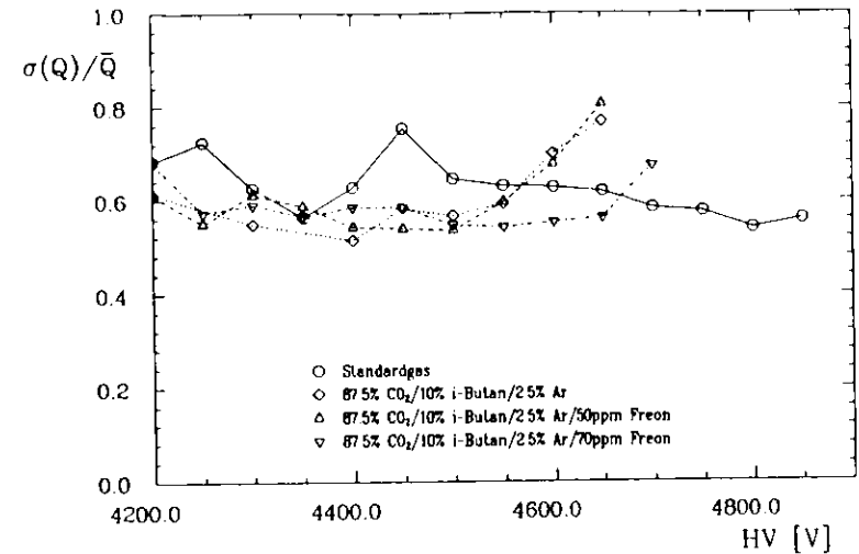
Abbildung 6.7: Relative Breiten der Ladungsverteilungen aller Pulse über 50mV in Abhängigkeit von der Hochspannung
