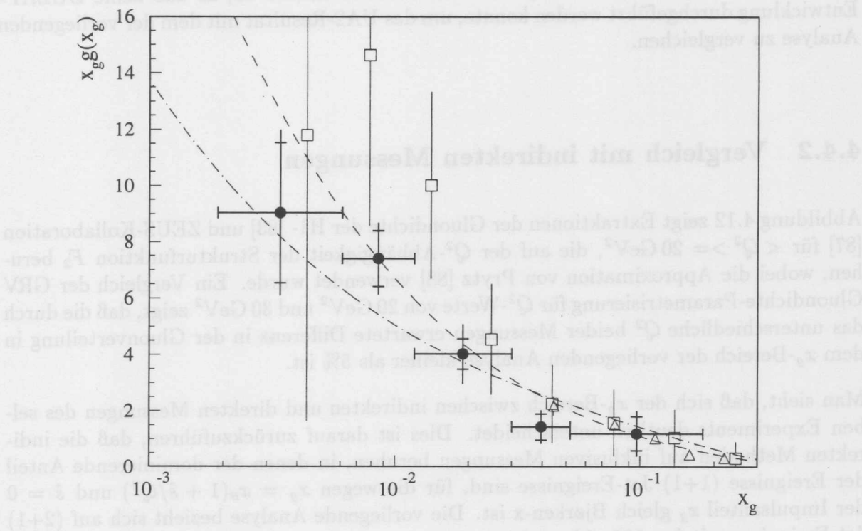
Abbildung 4.11: Vergleich der Gluonverteilung der vorliegenden Analyse (•) mit einer vorläufigen Messung der ZEUS Kollaboration (□) und einer mit den DGLAP-Gleichungen auf \langle Q^2 \rangle = 30 \text{ GeV}^2 transformierten Messung der NMC Kollaboration (Δ). Die Kurven sind die LO GRV'94 (---) und LO CTEQ3L (- · - ·) Parametrisierungen der Gluonverteilung.
