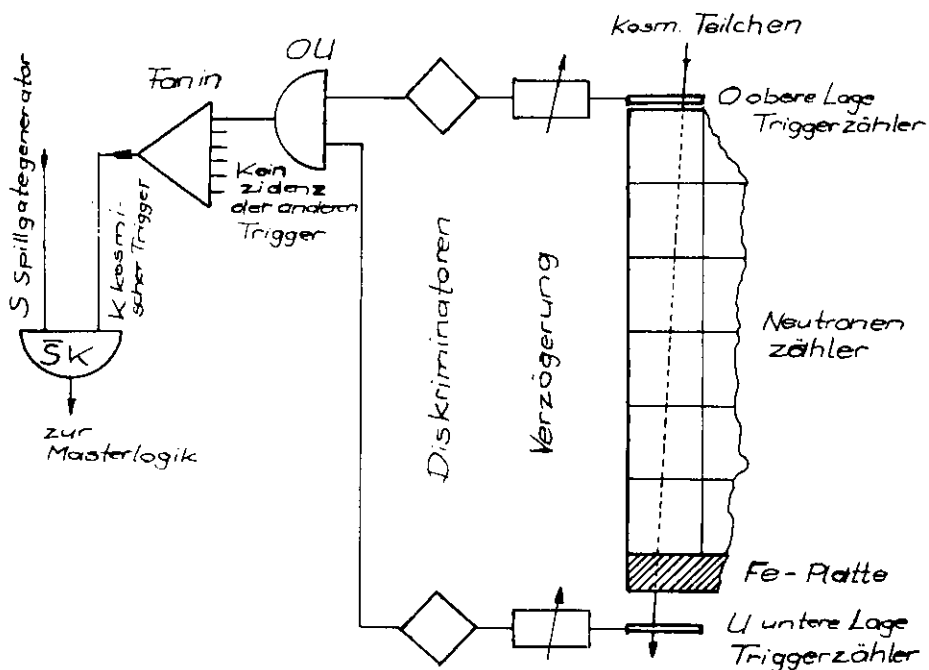
Abb.11 Logik der Triggerzähler für die Aufnahme von Impulshöhenspektren der kosmischen Strahlung
