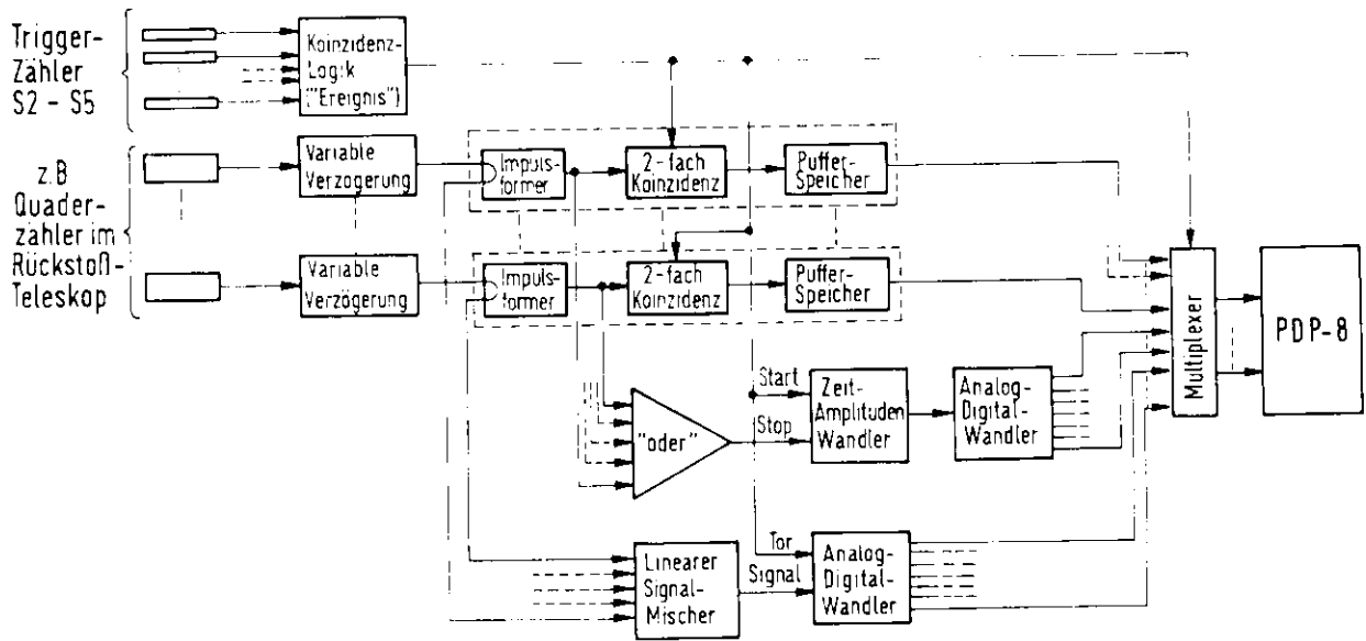
Abb.10 Prinzip der elektronischen Einzelereignis-Registrierung dargestellt am Beispiel der Quaderzähler im Rückstoßteleskop.
