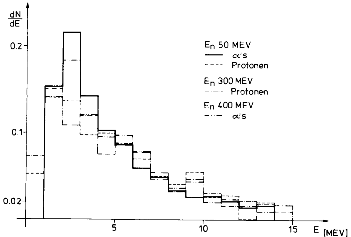
Abb. 17 c) Energiespektrum der Evaporationsteilchen nach Bertini 24 für Neutronen mit E_n kin. Energie auf C^{12}
