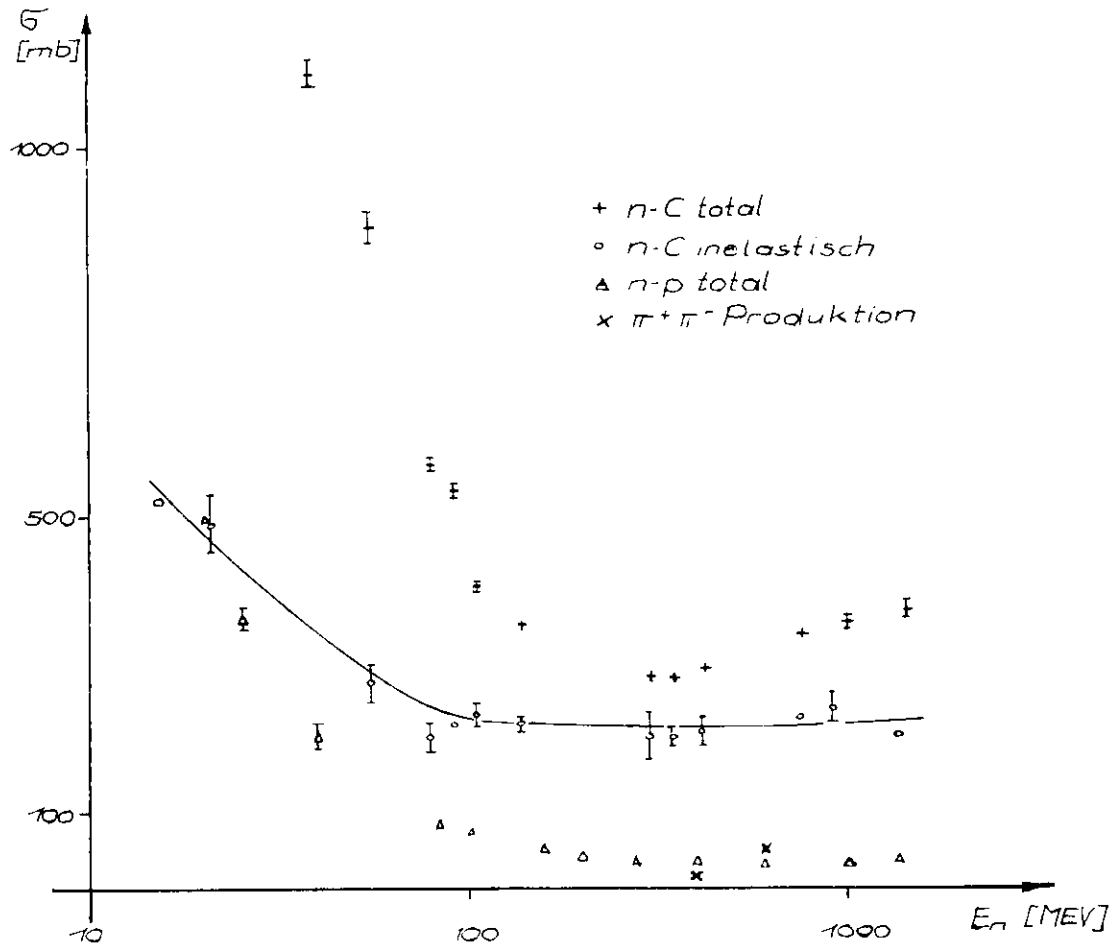
Abb.18 Wirkungsquerschnitte für n-p und n-C Streuung; durchgezogene Linie: angepaßte Funktion (III.12)
