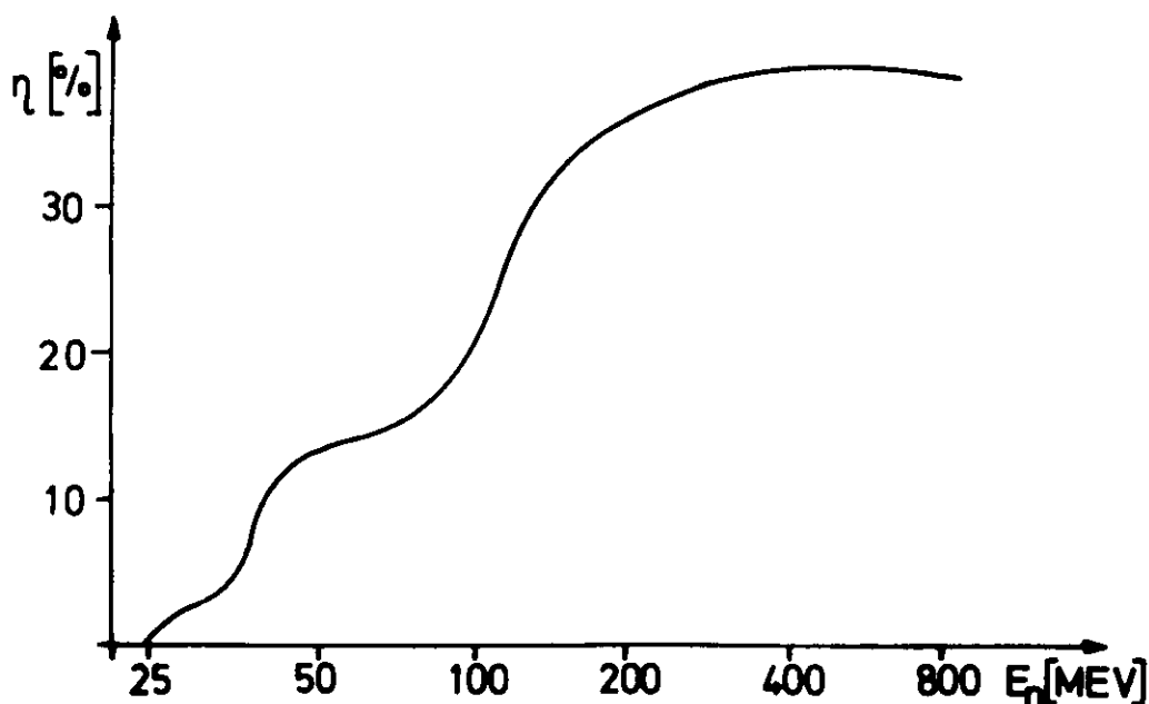
Abb.15 n(E_n) berechnet mit dem Programm von Kurz 1) , S = 20 MeV, Zählergröße 60 \times 60 \times 50 cm 3 gesetzt, Energiebereich erweitert.
