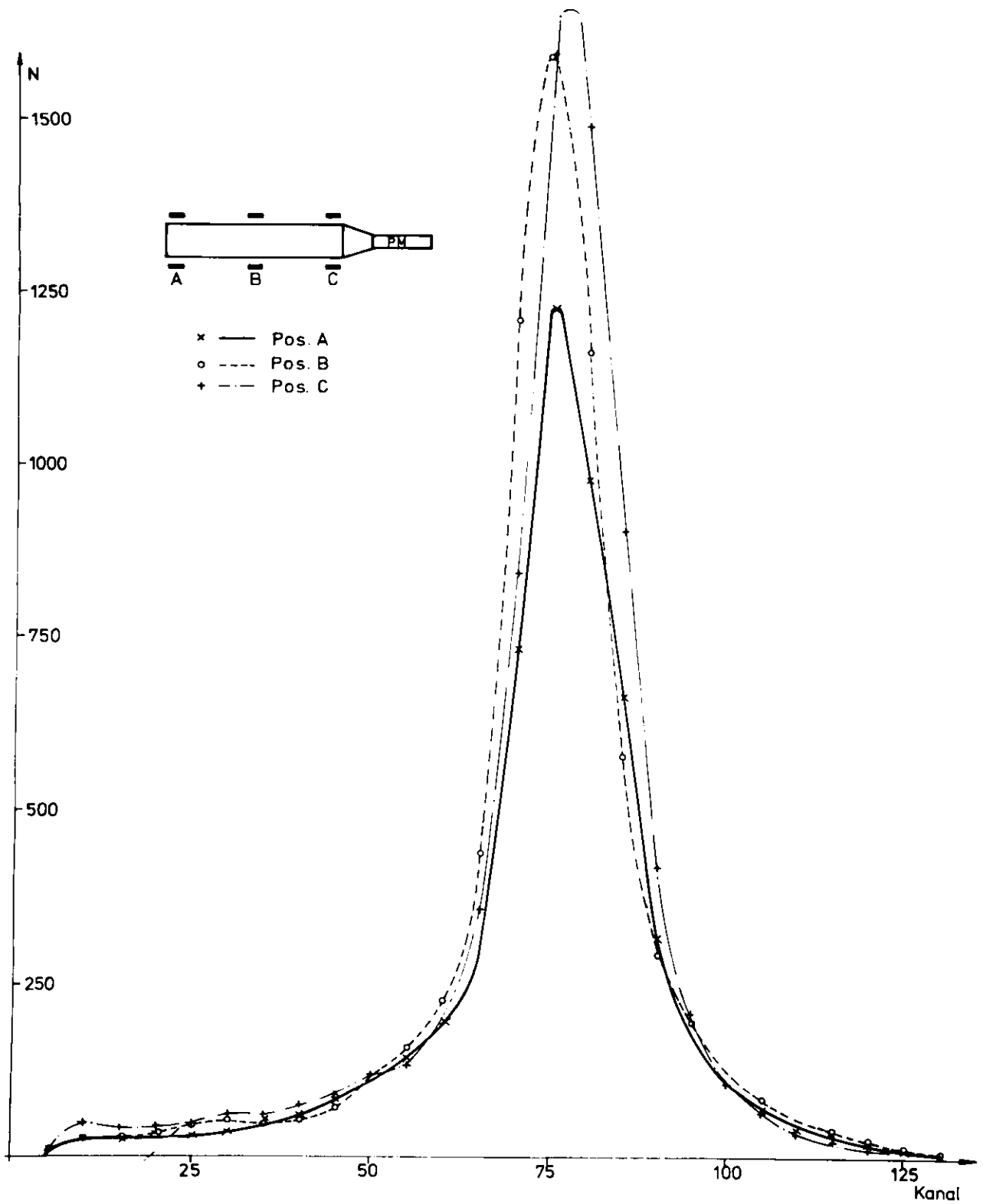
Abb. 5 Impulshöhenspektren kosmischer Strahlung an 3 Stellen des Zählers gleichzeitig aufgenommen
