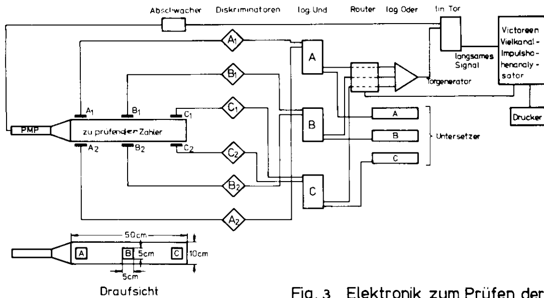
Fig. 3 Elektronik zum Prüfen der Zähler mit Höhenstrahlen
