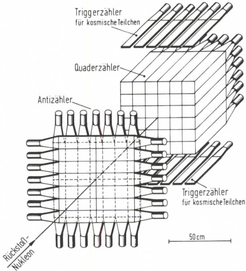
Abb.1 Szintillationszähler des Rückstoßteleskops (Schematische Explosivzeichnung)
