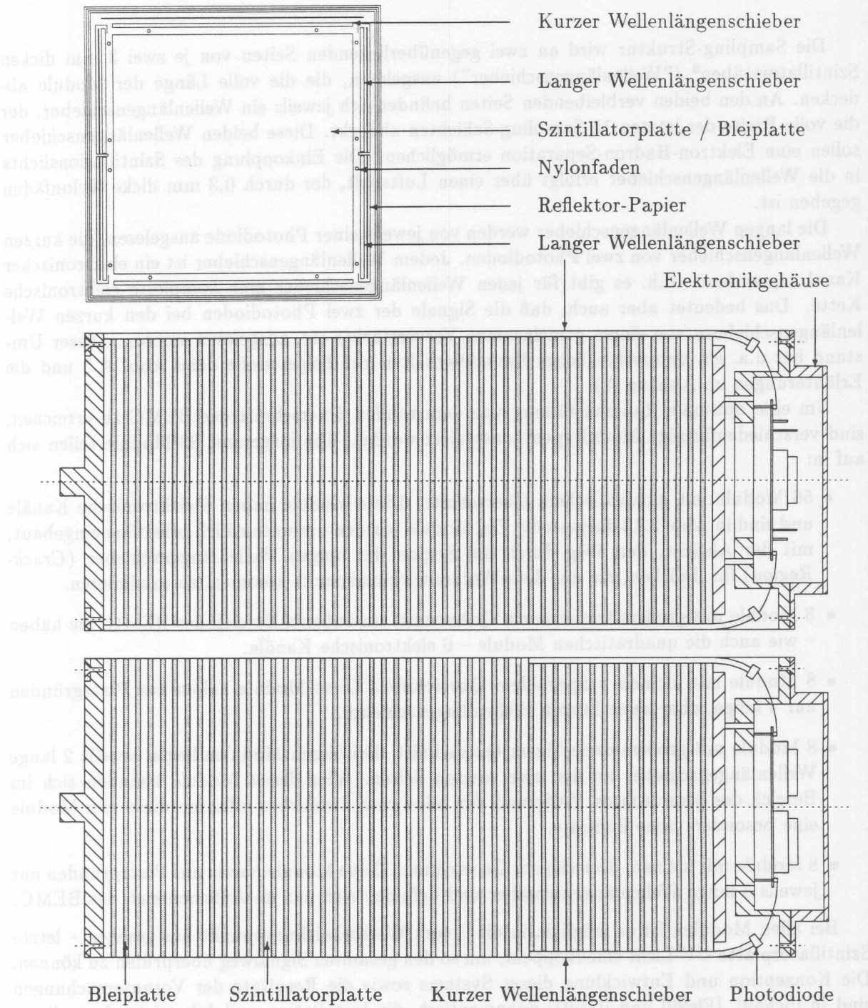
Abb. 3.13: Schnitt durch ein BEMC-Modul mit quadratischem Querschnitt Die schattierten Bereiche kennzeichnen die Bleiplatten, die sich mit Szintillatorplatten abwechseln. Die langen Wellenlängenschieber grenzen an alle Szintillatorschichten (oben abgebildet), während die kurzen Wellenlängenschieber nur an den hinteren 15 Schichten anliegen. Auf den Stirnflächen der Wellenlängenschieber sind Photodioden aufgeklebt, deren Signale von ladungsempfindlichen Vorverstärkern, die im Elektronikgehäuse untergebracht sind, verarbeitet werden.
