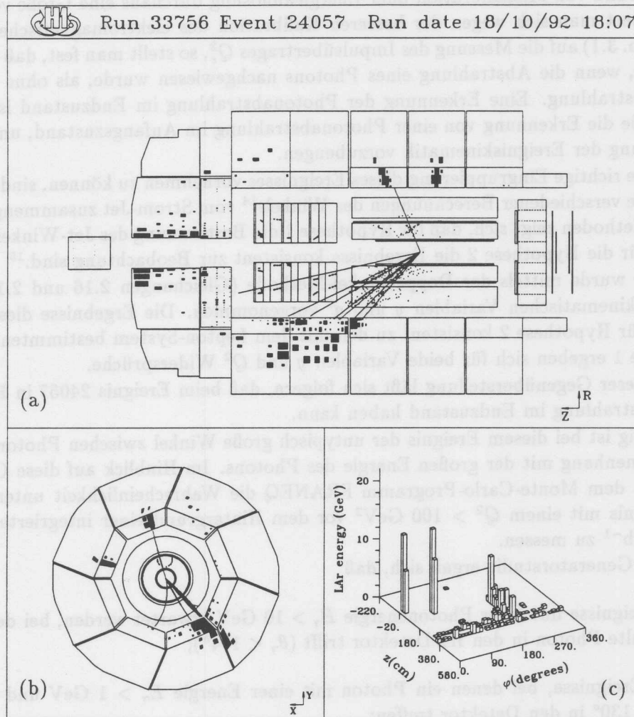
Abb. 4.14: Radiatives, tief inelastisches Ereignis mit hohem Q^2 Zur Kinematik dieses Ereignisses siehe Tab. 4.1.
