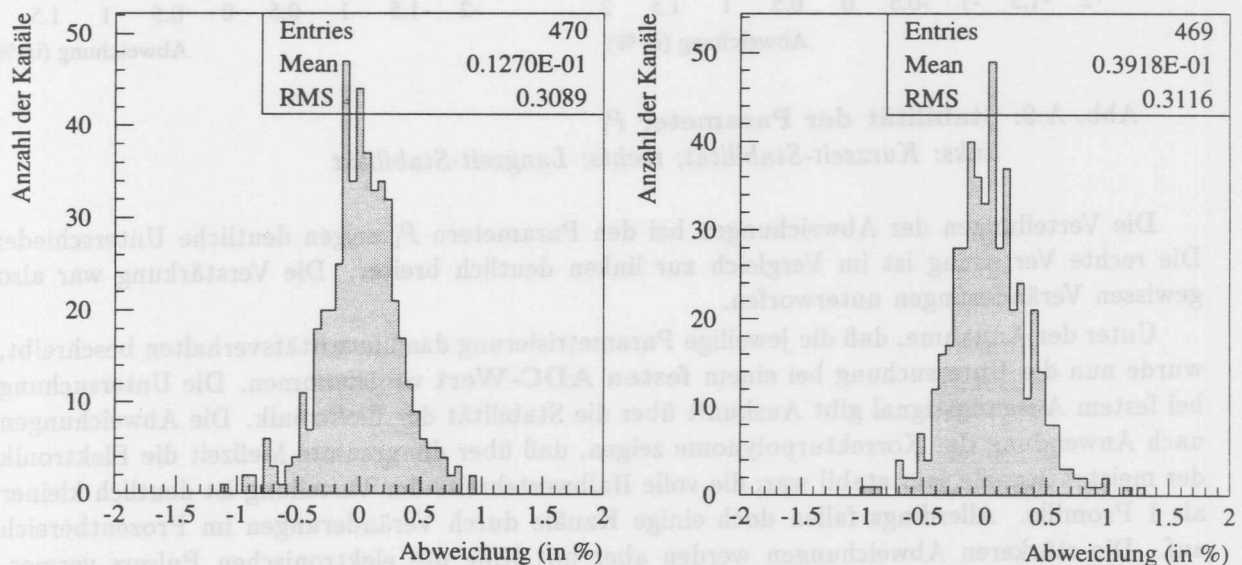
Abb. A.8: Stabilität der Pedestals
