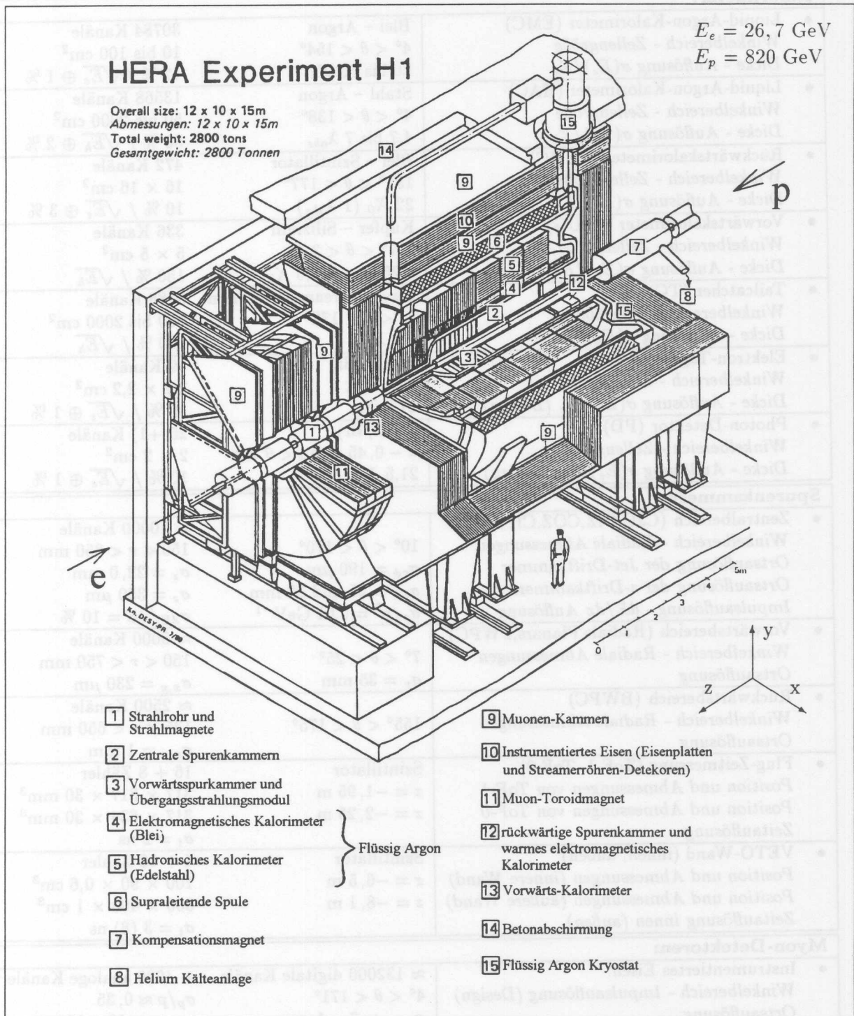
Abb. 3.2: Der H1-Detektor Perspektivische Darstellung aus [H1C86]
