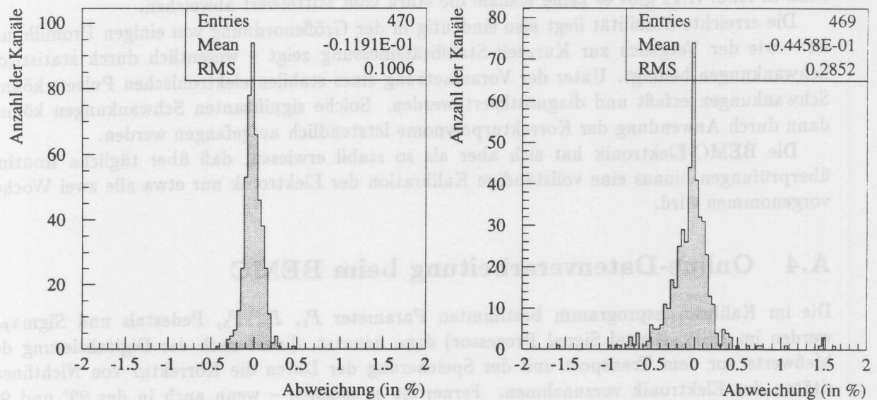
Abb. A.10: Stabilität der Elektronik bei 1500 ADC-Einheiten
