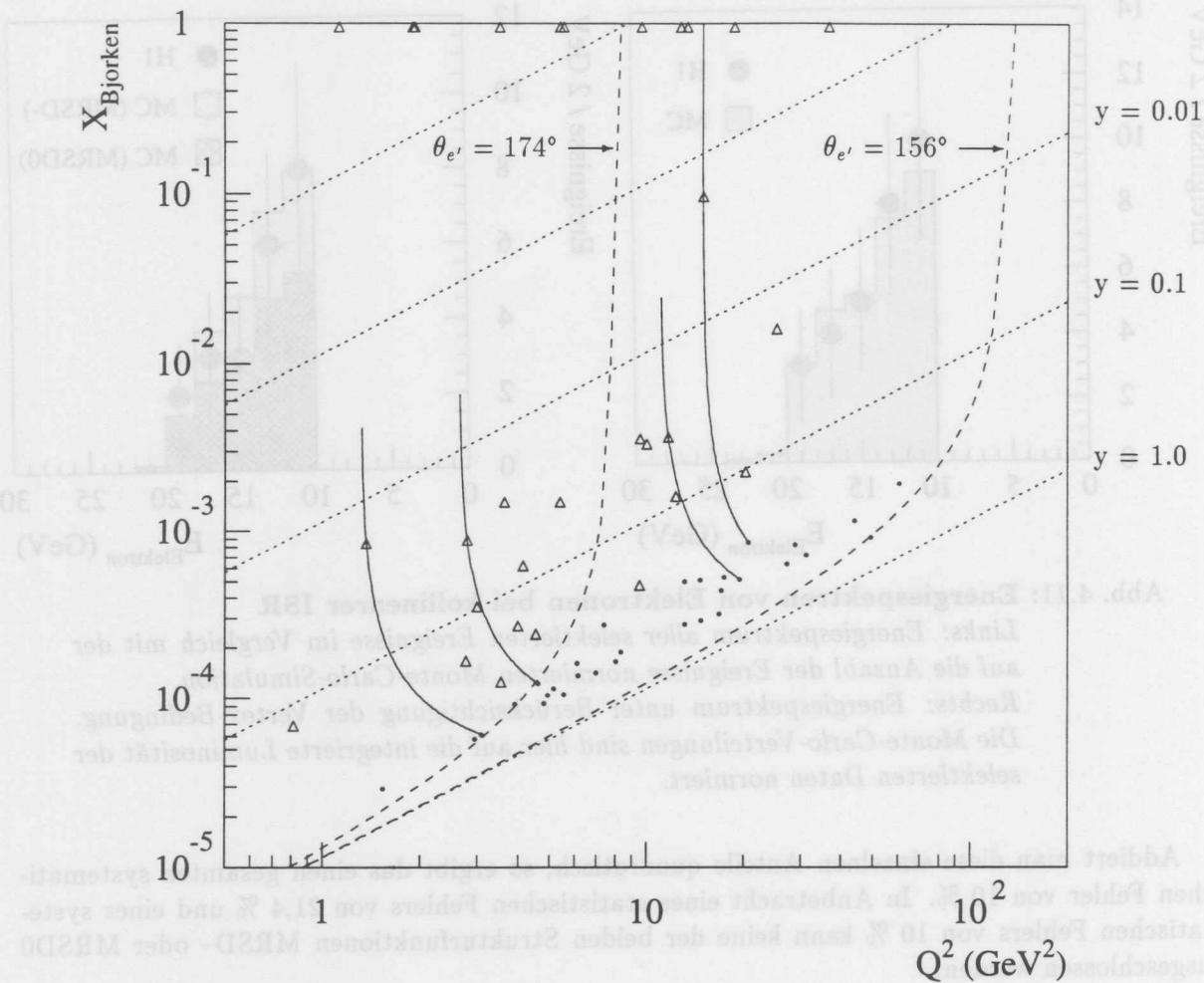
Abb. 4.12: Migration in der kinematischen Ebene durch kollineare ISR
