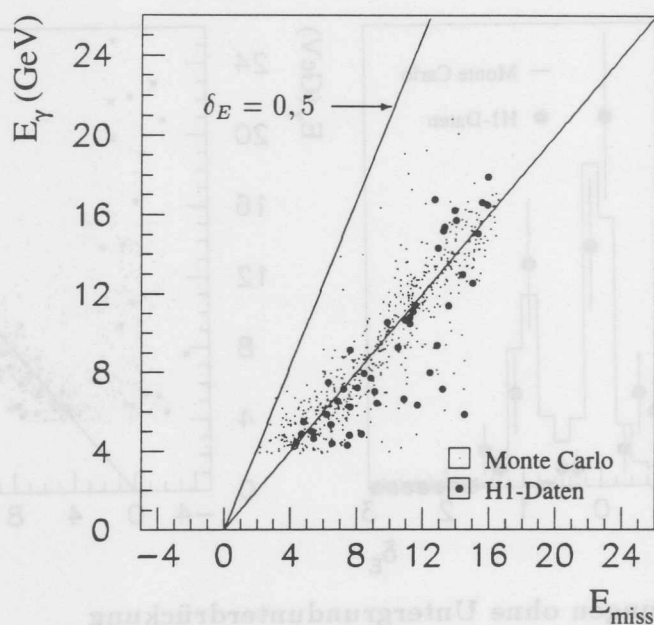
Abb. 4.6: Untergrundunterdrückung mit Hilfe von E_{ET} und E_{miss}
