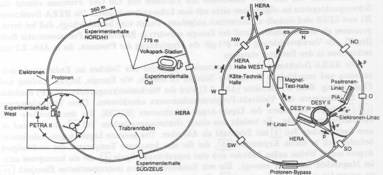
Abb. 3.1: Der Speicherring HERA und seine Vorbeschleuniger
