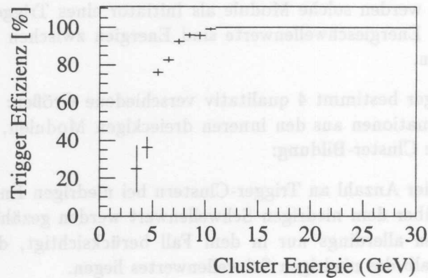
Abb. 3.16: Triggereffizienz für den energiereichsten Cluster im BEMC
