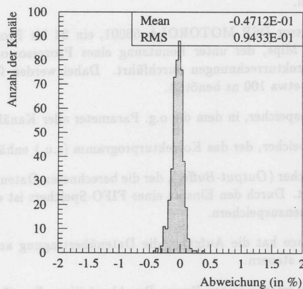
Abb. A.11: Stabilität der Energiemessung bei ca. 30 GeV
