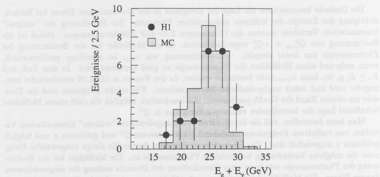
Abb. 4.13: Summenspektrum gebildet aus Elektron- und Photonenergie
