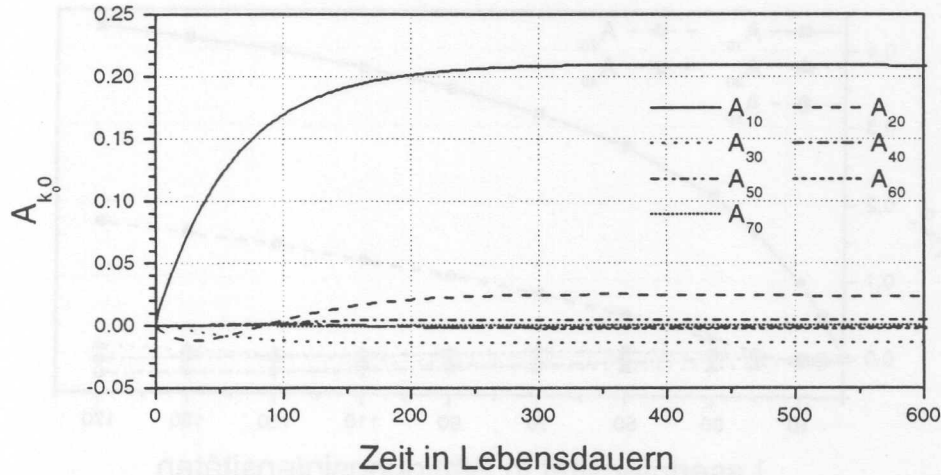
Abbildung 2.3: Zeitliche Entwicklung der Multipolmomente bei zirkularer polarisation des Laserlichts. Die Zeit ist in Einheiten der Lebensdauer \tau angegeben. Der Laser ist auf den Schwerpunkt des Multipletts abgestimmt mit einer Intensität von I_0 = 30I_{\text{sat}} . Die Depolarisationsrate beträgt \tau_{\text{depol}} = 0.01\tau .
