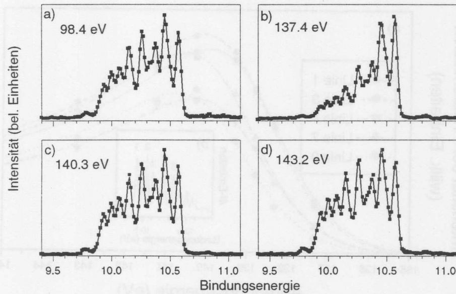
Abbildung 6.8: Europium 4f^{-1} -Photoelektronenspektren bei vier verschiedenen Anregungsenergien im Bereich der Riesenresonanz.
