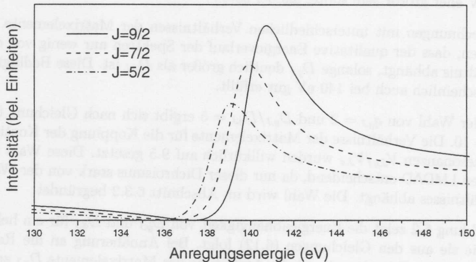
Abbildung 6.3: Intensitäten |D_{gJ}|^2 für unterschiedliche Werte von J . Die Resonanzpositionen unterscheiden sich um etwa 0.8 eV. Das Verhältnis der Intensitäten entspricht den Multiplizitäten.
