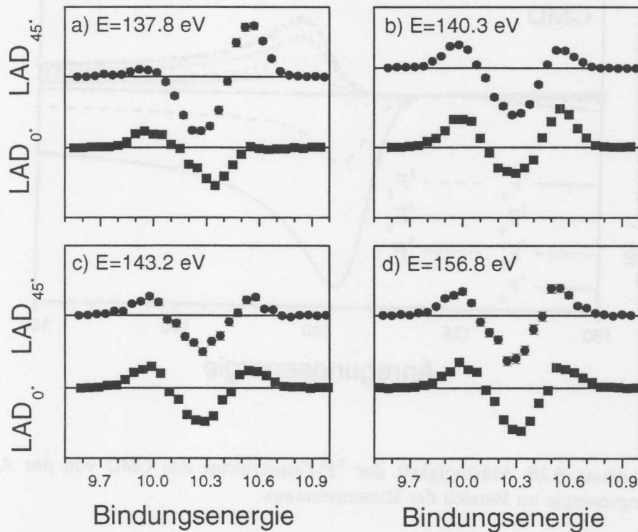
Abbildung 6.15: Experimenteller LAD bei vier verschiedenen Anregungsenergien im Bereich der Riesenresonanz.
