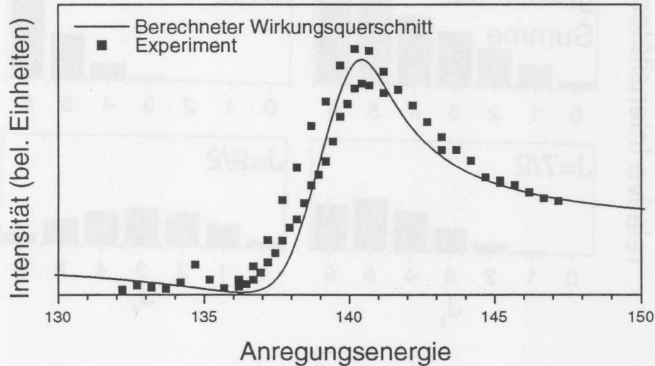
Abbildung 6.4: Vergleich der Energieabhängigkeit des berechneten totalen 4f^{-1} -Wirkungsquerschnitts mit den gemessenen Werten aus Abbildung 6.1.
