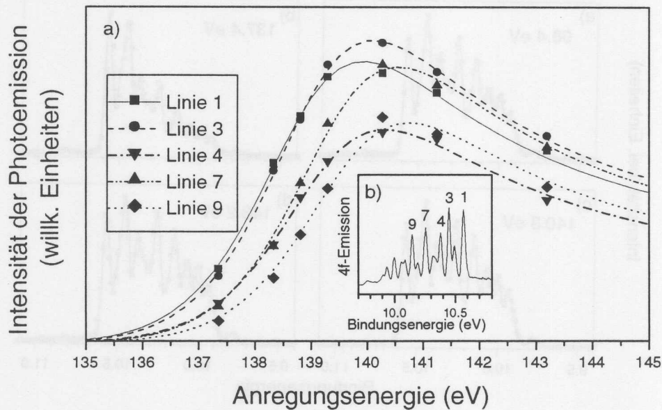
Abbildung 6.9: Relative Intensitäten der Eu 4f-Feinstrukturkomponenten an sieben Energiepositionen im Bereich der Riesenresonanz. Der Energieverlauf der Linien wurde mit Fanoprofilen angepasst. Die Parameter der Anpassung sind in Tabelle 6.1 angegeben.
