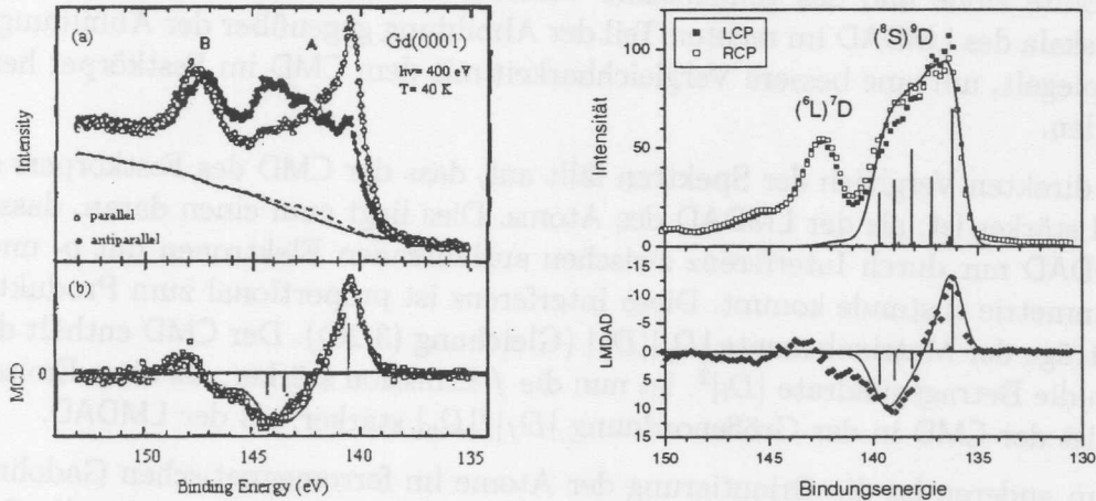
Abbildung 4.9: Vergleich des CMD an einer Gd Oberfläche [Are95](links) mit dem LMDAD von atomarem Europium (Abbildung 4.5). (Erläuterungen siehe Text.)
