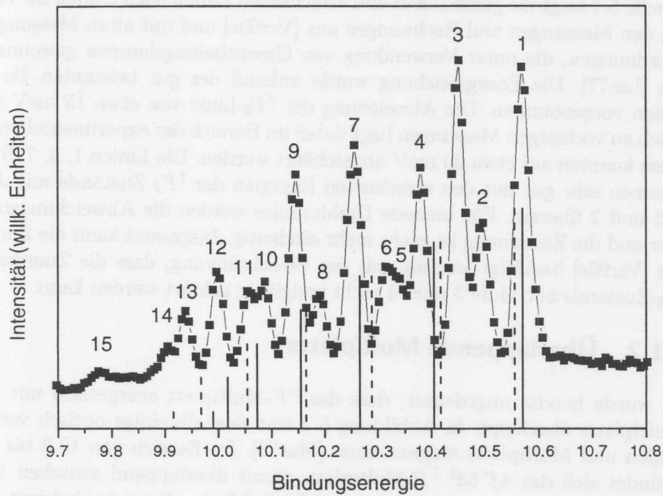
Abbildung 5.1: Europium 4f^{-1} -Photoionisationsspektrum. Die experimentelle Auflösung betrug 33 meV. Zum Vergleich wurden zwei {}^7F_J -Multipletts als Balkendiagramme eingezeichnet. Die durchgezogenen Balken entsprechen der Rechnung aus Tabelle 5.1. Die gestrichelten Balken geben die Rechnung aus [Ver99c] wieder, bei denen der Spin-Bahn-Parameter auf 95% reduziert wurde.
