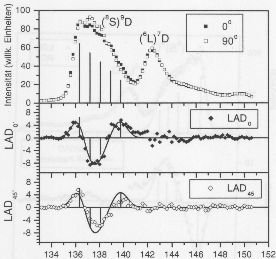
Abbildung 4.6: LAD der Europium 4d^{-1} -Photoionisation.
