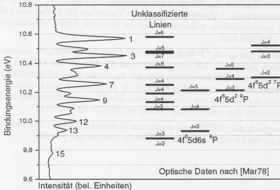
Abbildung 5.2: Das gemessene Europium 4f Photoelektronenspektrum (links) im Vergleich zu optisch vermessenen Energieniveaus aus [Mar78].
