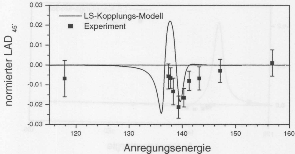
Abbildung 6.20: Feinstrukturintegrierter normierter LAD_{45^\circ} . Vergleich von Modell und Experiment.
