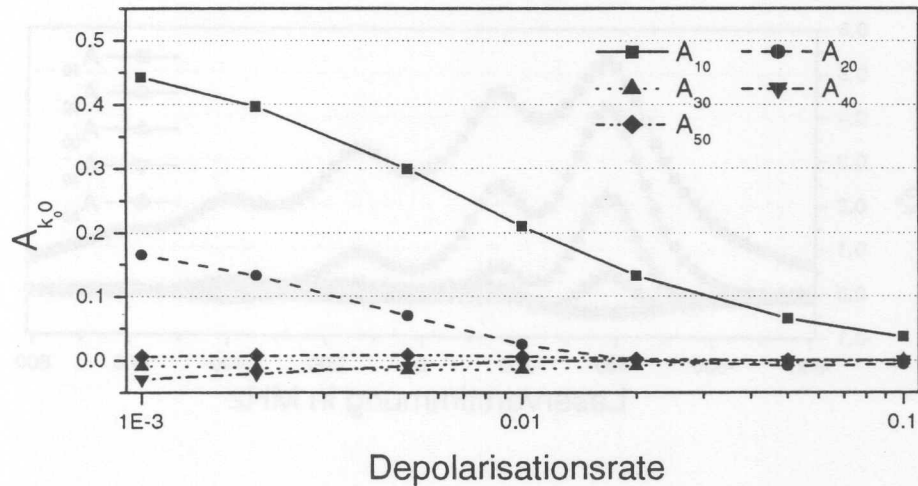
Abbildung 2.5: Abhängigkeit der Multipolmomente von der Depolarisation \tau_{\text{depol}} . Der Laser ist auf den Schwerpunkt des Multipletts abgestimmt mit einer Intensität von I_0 = 30I_{\text{sat}} . Das Laserlicht ist zirkular polarisiert. Angegeben sind die Multipolmomente nach einer Pumpdauer von 400\tau
