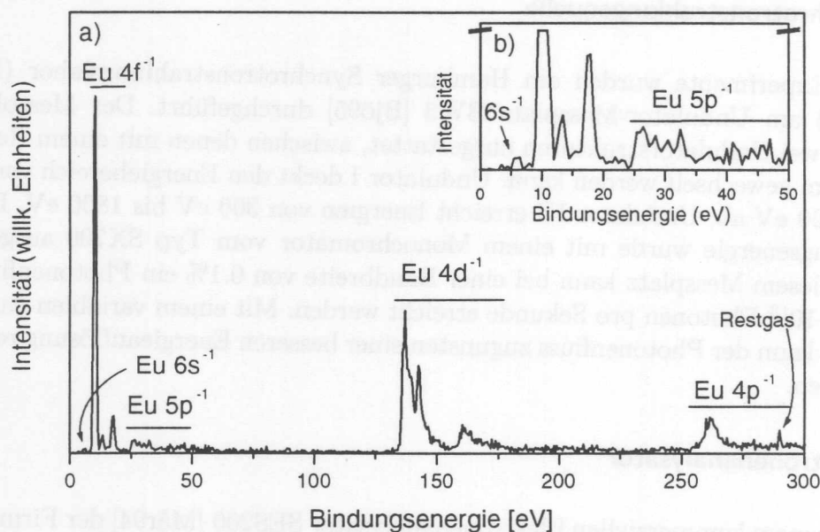
Abbildung 3.4: Übersichtsspektrum über die Photoelektronenemission atomaren Europiums bei einer Anregungsenergie von 455 eV. Die markierten Strukturen sind im Text erläutert. Das Spektrum wurde nicht um die energieabhängige Transmission des Analysators korrigiert. Die relativen Intensitäten der Linien sind daher nicht Aussagekräftig.
