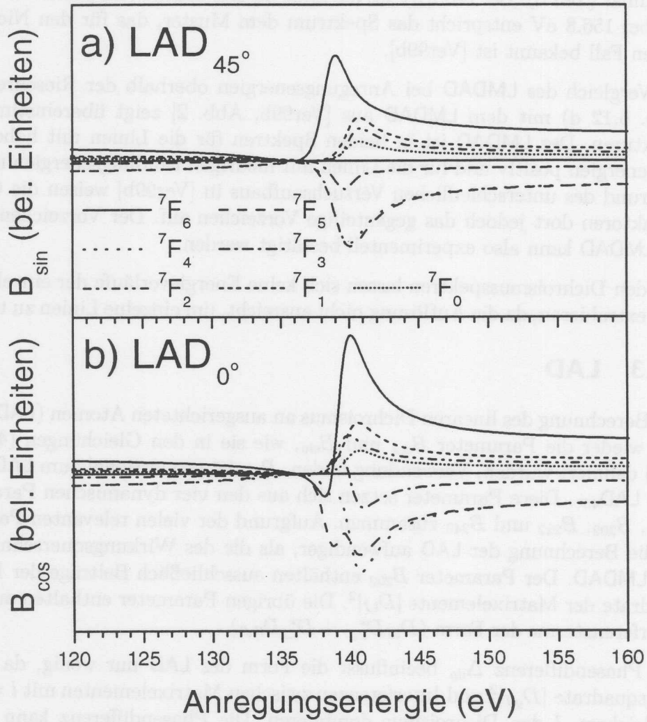
Abbildung 6.13: Abhängigkeit der {}^7F -Feinstruktur des LAD von der Anregungsenergie im Bereich der Riesenresonanz.
