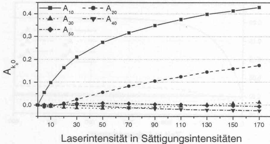
Abbildung 2.4: Abhängigkeit der Multipolmomente von der Intensität des Lasers I_0/I_{\text{sat}} . Der Laser ist auf den Schwerpunkt des Multipletts abgestimmt und zirkular polarisiert. Angegeben sind die Multipolmomente nach einer Pumpdauer von 400\tau . Die Depolarisationsrate wurde als 0.01\tau angenommen.
