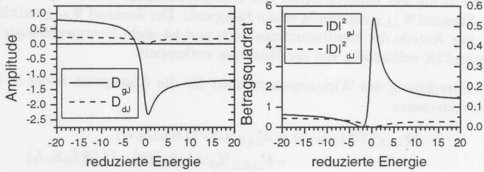
Abbildung 6.2: Links: Die Abhängigkeit der Matrixelemente D_{gJ} und D_{dJ} von der reduzierten Energie \epsilon .
