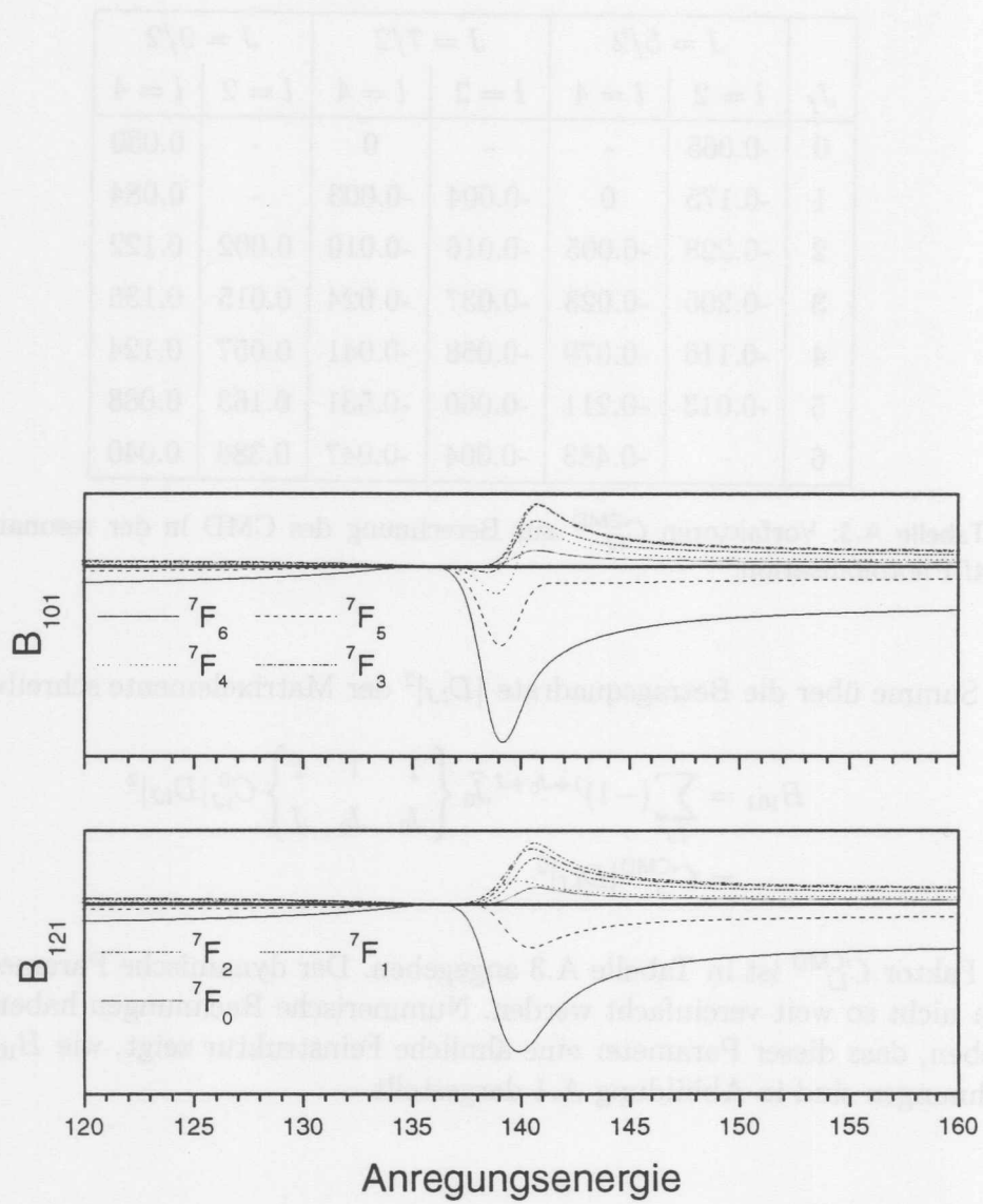
Abbildung A.1: Vergleich der dynamischen Parameter B_{121} und B_{101} .
