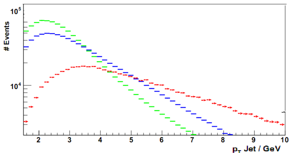
Слика 2.5.5 Илустрација облика дистрибуција трансверзалног импулса млазева који потичу од кваркова различитих аромета: лаки кваркови (зелена), с кварк (плава) и b кварк (црвена).
