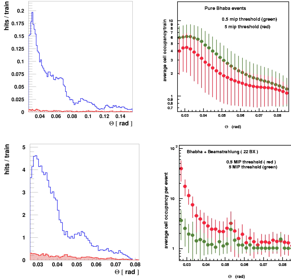
Слика 1.3.13 Ангажованост система за читавање а) од сигнала и физичког фона за ( R\phi ) сегментацију, интегрисаног по возу банчева б) од сигнала и физичког фона за тракасту сегментацију ц) и д) од сигнала са и без присуства машинског фона за ( R\phi ) сегментацију.
