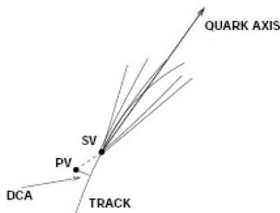
Слика 2.3.6 Дефиниција параметра судара: најкраће растојање трага од примарног вертекса у r\varphi равни.
