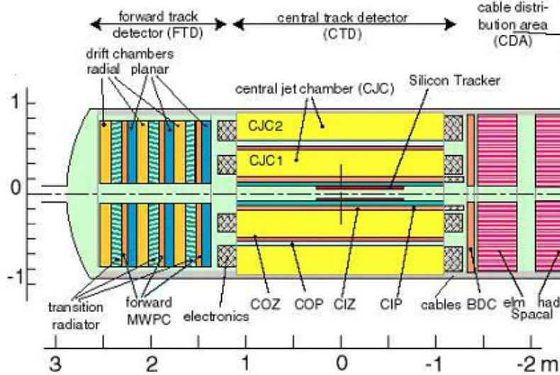
Слика 2.2.3 Попречни пресек ( r_z равн) система за реконструкцију трагова. На слици је приказан предњи и централни део система за реконструкцију трагова са поддетекторским системима.
